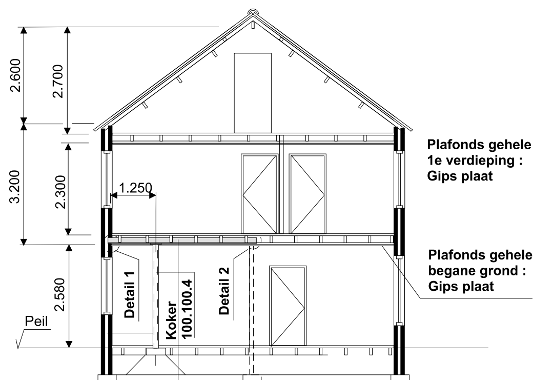
Doorsnede A - A Gewijzigde situatie
