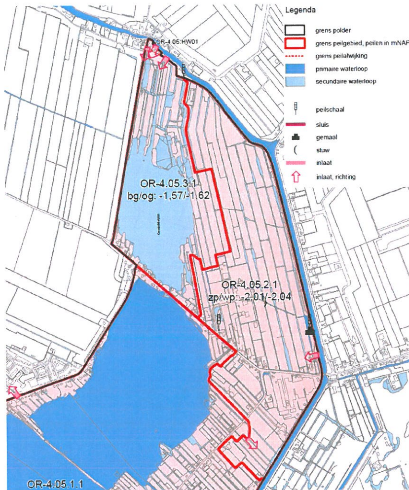
Figuur 5. Toekomstige waterhuishoudkundige situatie Geerpolder
