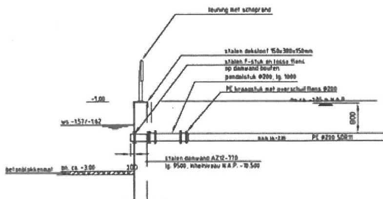
doorsnede uitstroominlaat schaal 1:50
