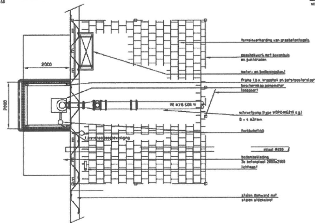
bovenaanzicht instroomzijde schaal 1:50
