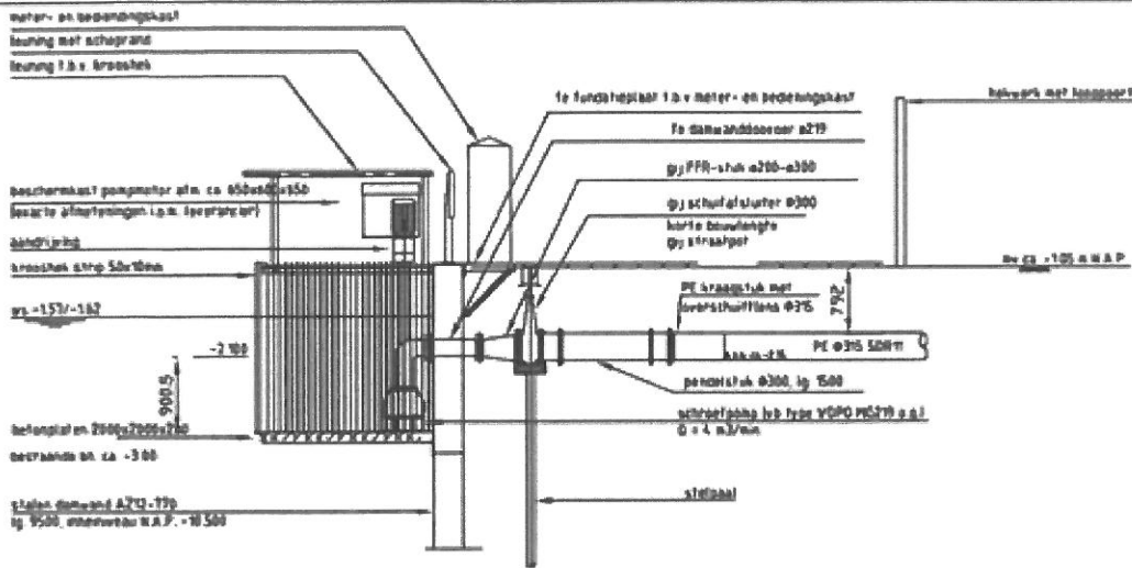
doorsnede pompput schaal 1:50
