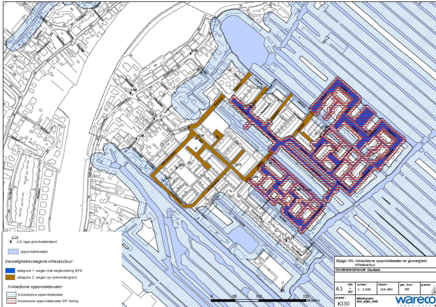
Tekening 9 Invloedsfeer oppervlaktewater
