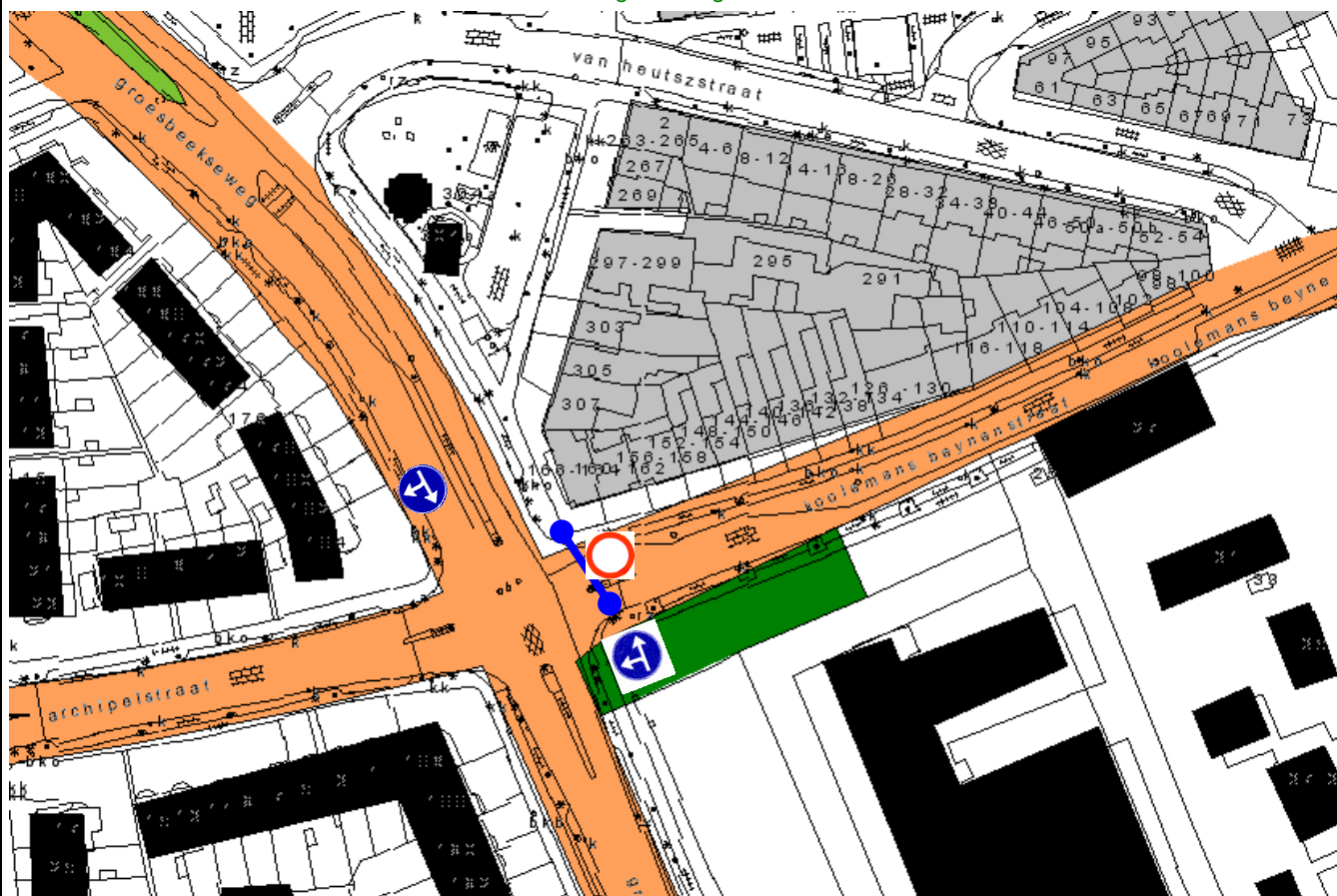
Situatietekening 6
