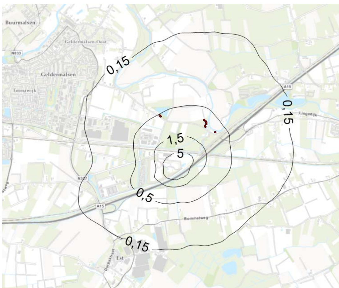
Figuur 5.1 Geurconcentratie in de omgeving als gevolg van de vergunde situatie van Avri. Gepresenteerd zijn van buiten naar binnen de geurcontouren van 0,15 / 0,5 / 1,5 en 5 \text{ouE}/\text{m}^3 als 98-percentiel.
