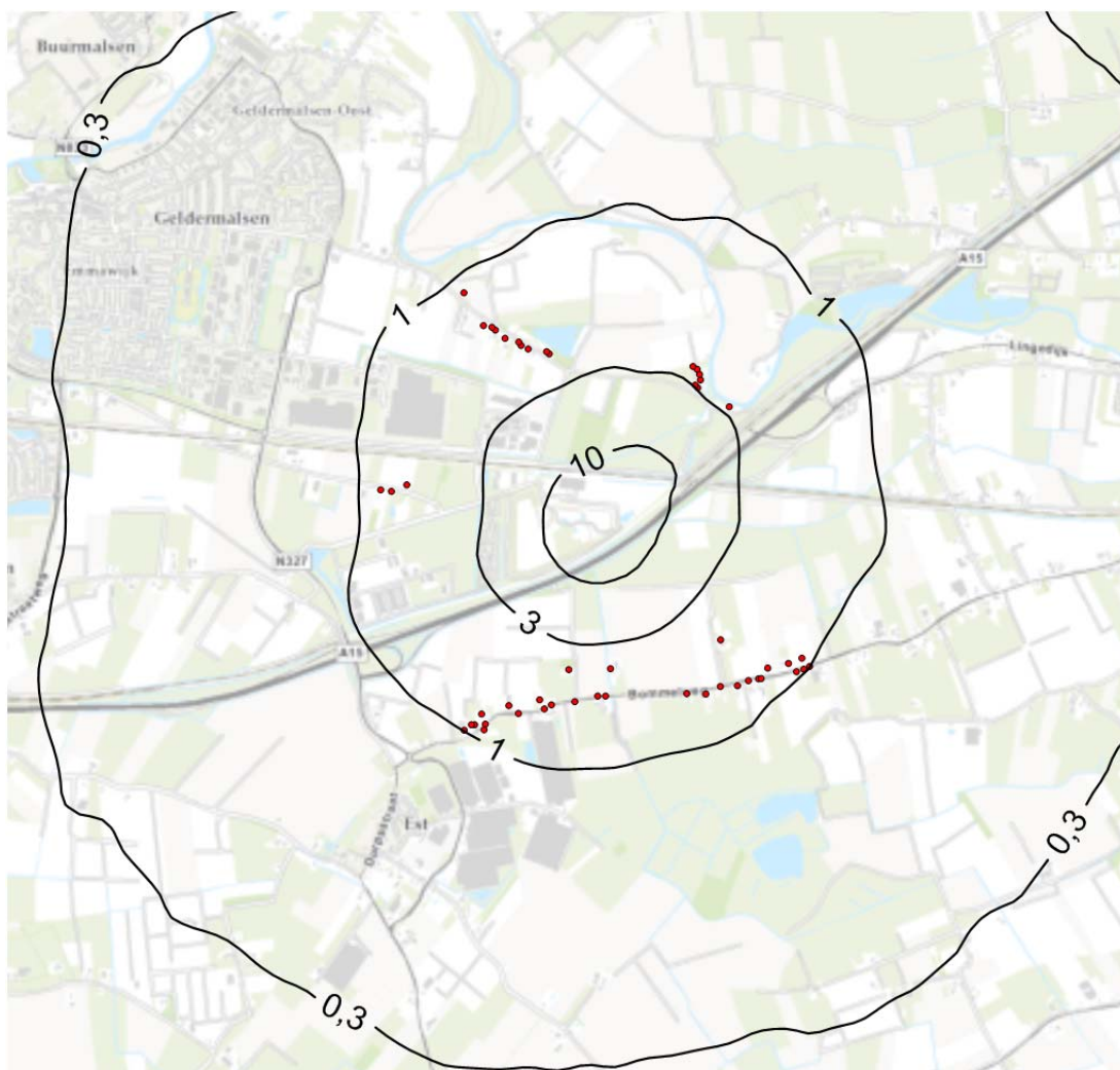
Figuur 4.2 Geurconcentratie in de omgeving als gevolg van de voorgenomen activiteiten van Avri. Gepresenteerd zijn van buiten naar binnen de geurcontouren van 0,3 / 1 / 3 en 10 ou_E/m^3 als 99,5-percentiel.
