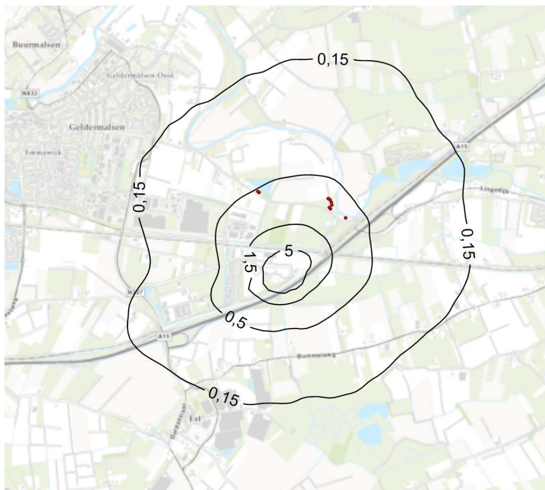
Figuur 4.1 Geurconcentratie in de omgeving als gevolg van de voorgenomen activiteiten van Avri. Gepresenteerd zijn van buiten naar binnen de geurcontouren van 0,15 / 0,5 / 1,5 en 5 ou_E/m^3 als 98-percentiel.
