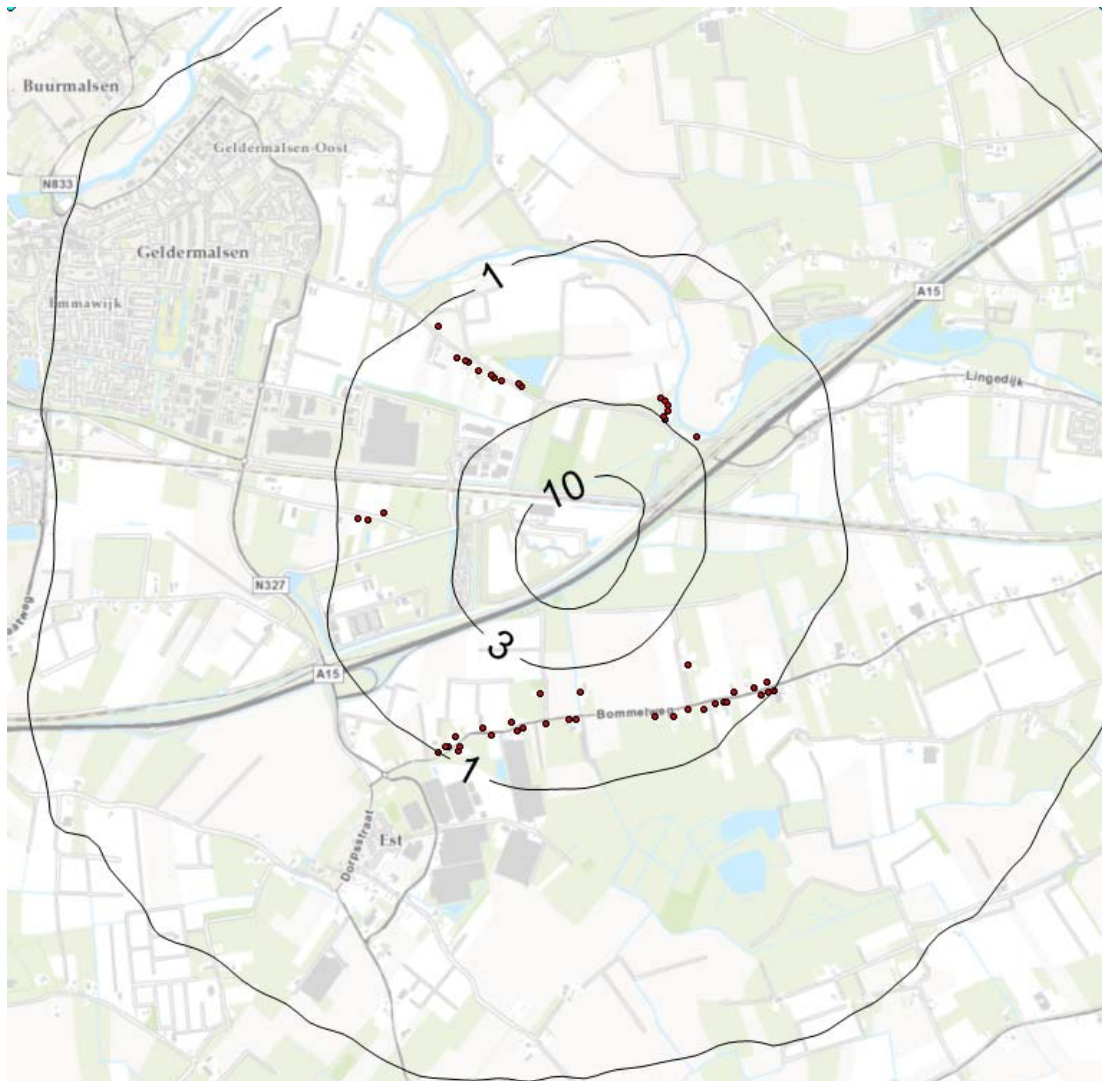
Figuur 5.2 Geurconcentratie in de omgeving als gevolg van de vergunde situatie van Avri. Gepresenteerd zijn van buiten naar binnen de geurcontouren van 0,3 / 1 / 3 en 10 ou_E/m^3 als 99,5-percentiel.
