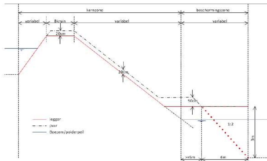
Figuur 2: Zoning van de waterkering
