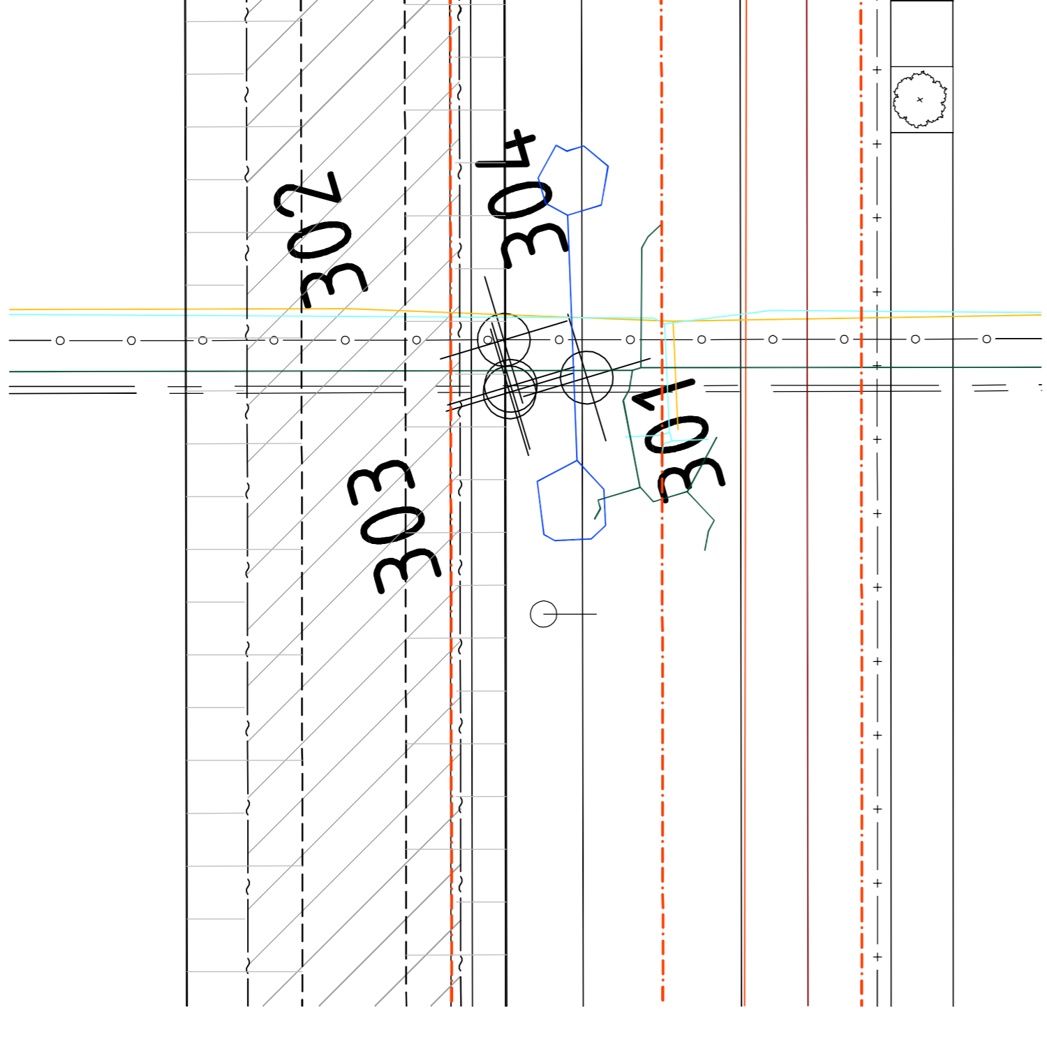
DETAIL SCHAAL 1:200
