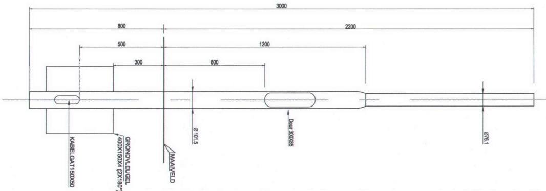
MA 28 Schaal 1:10
