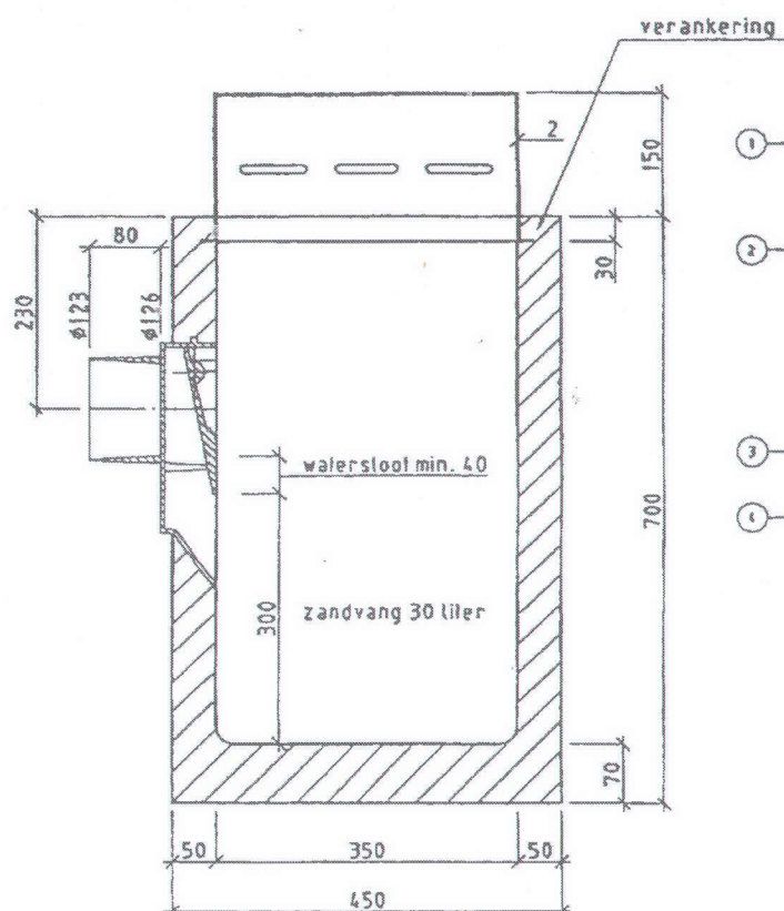
doorsnede A
