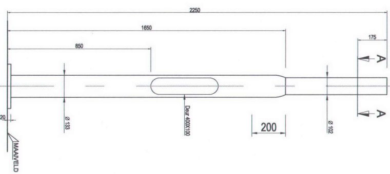
MA 50 met Voetplaat Schaal 1:10
