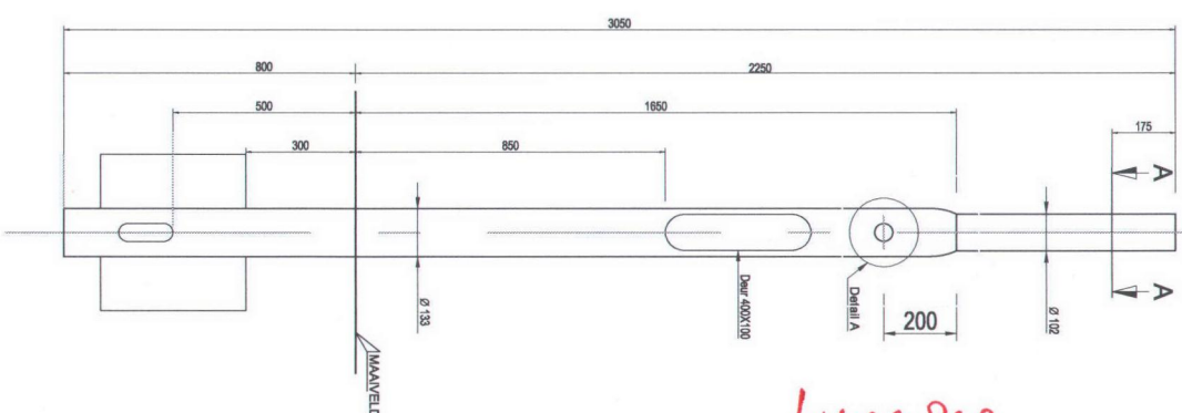
MA 50 met Drukknop Schaal 1:10
