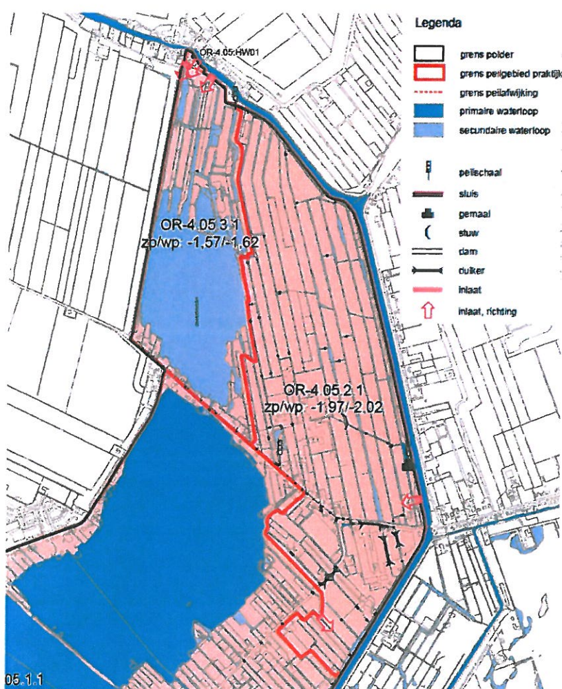
Figuur 2. Huidige waterhuishoudkundige situatie Geerpolder
