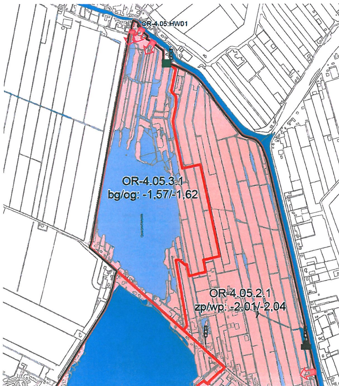
Figuur 3: De gemaalallocatie van gemaal Geerpolder is weergegeven met het groene vierkant
