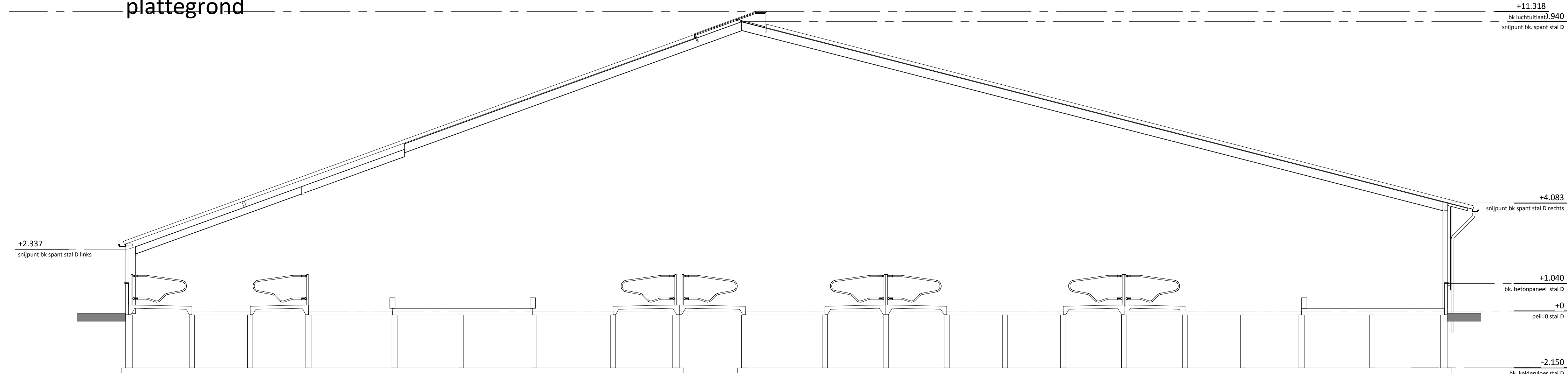
doorsnede D-D
