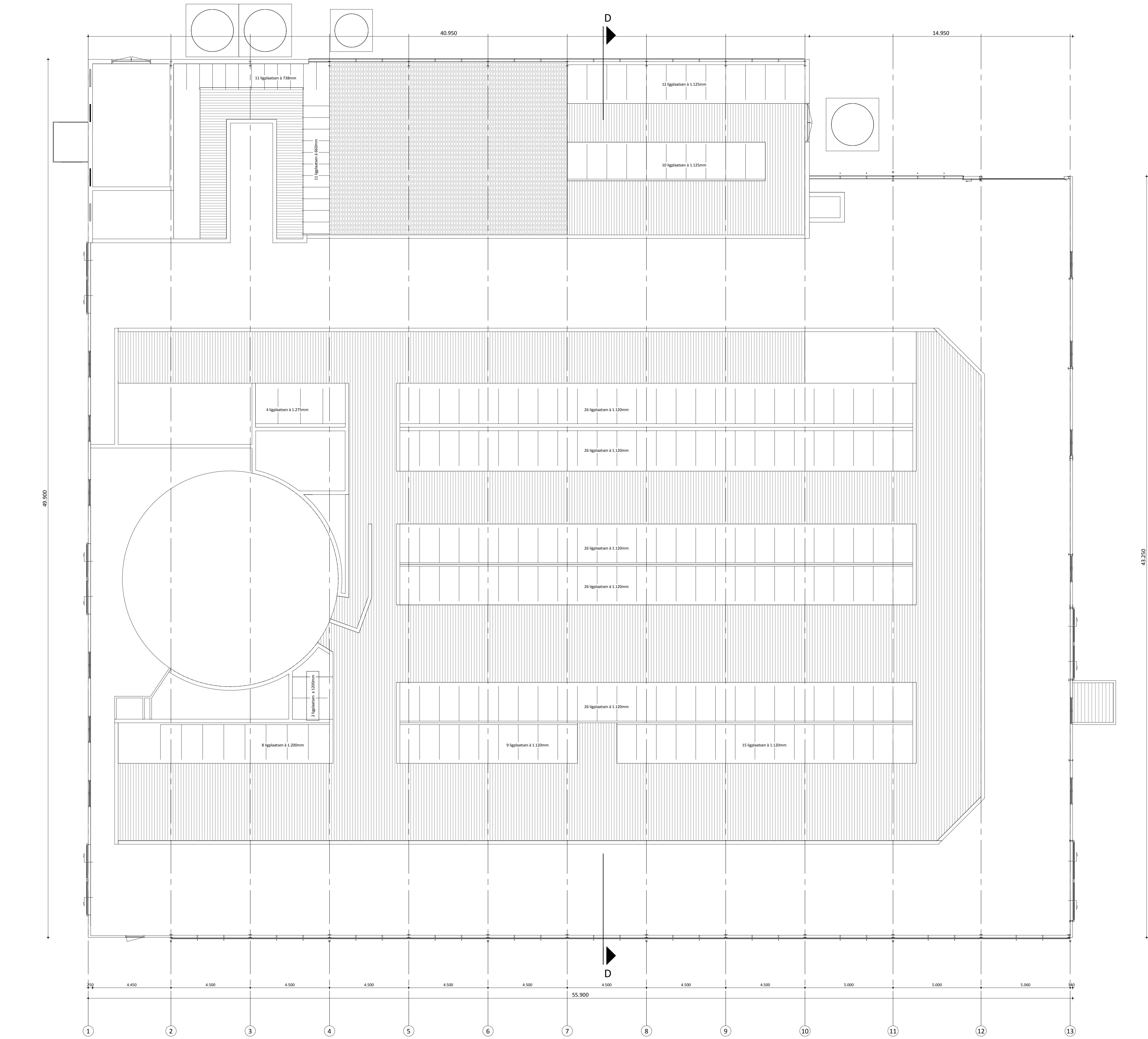
plattegrond
