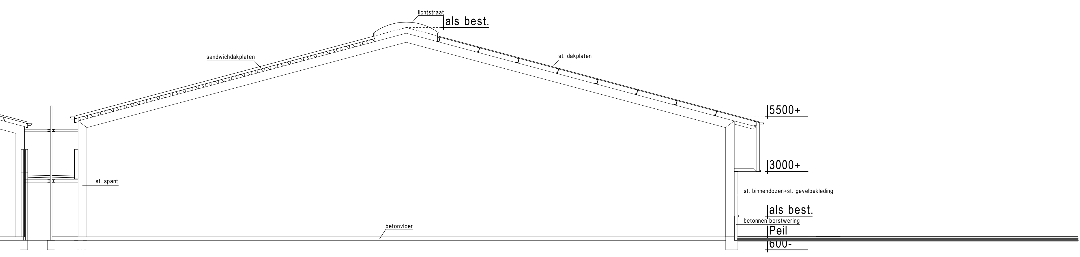
doorsnede bedrijfsruimte
