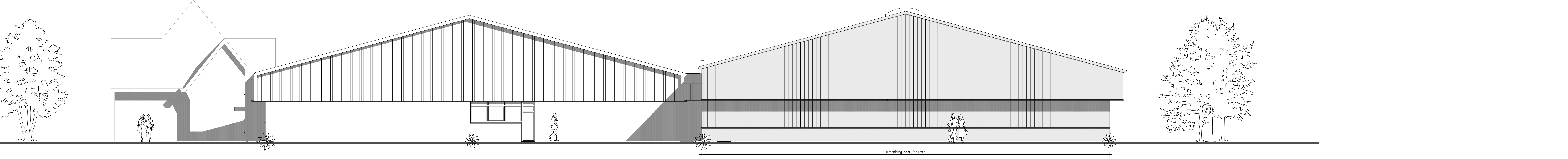
r. zijgevel
