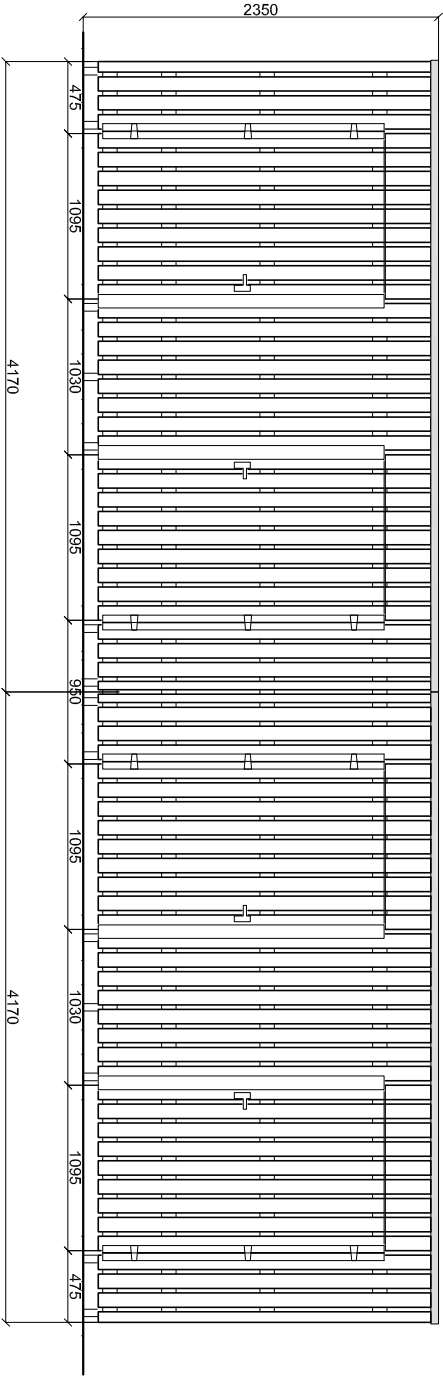
voorraanzicht
