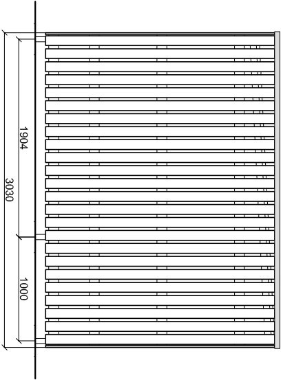
zijaanzicht
