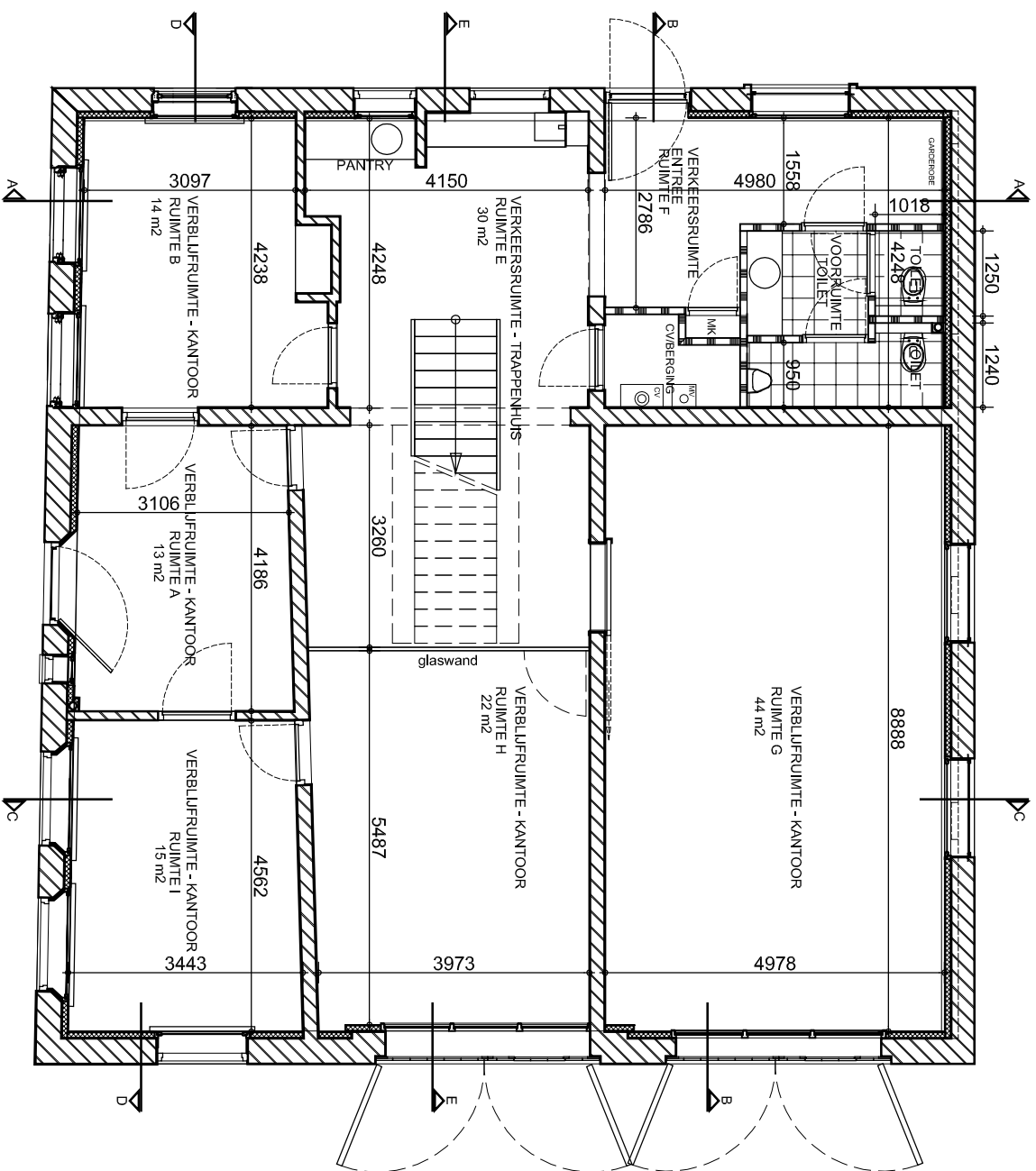
PLATEGROND BEGANEGROND
