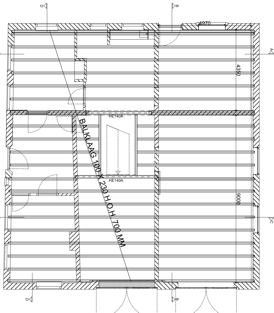
BALKAAG 1E VERDIEPINGSVLOER
