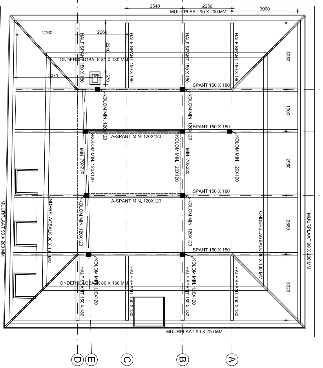
OVERZICHT SPANTEN OP 1E VERDIEPINGSVLOER
