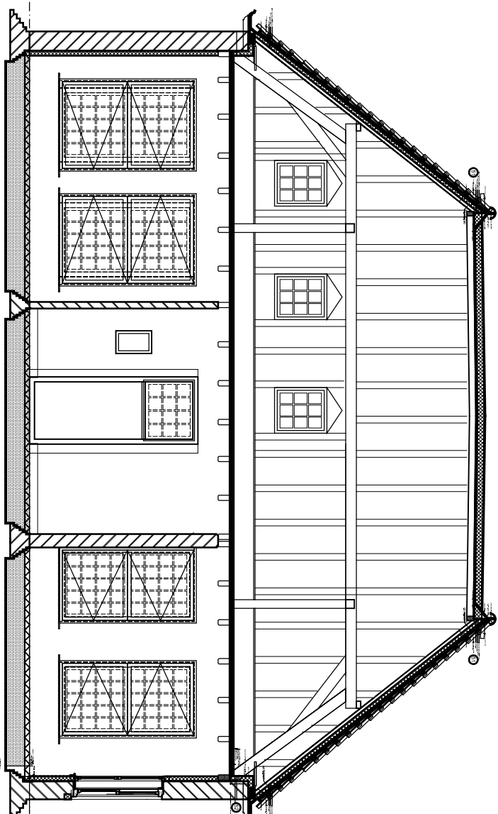
DOORSNEDE / AANZICHT D-D
