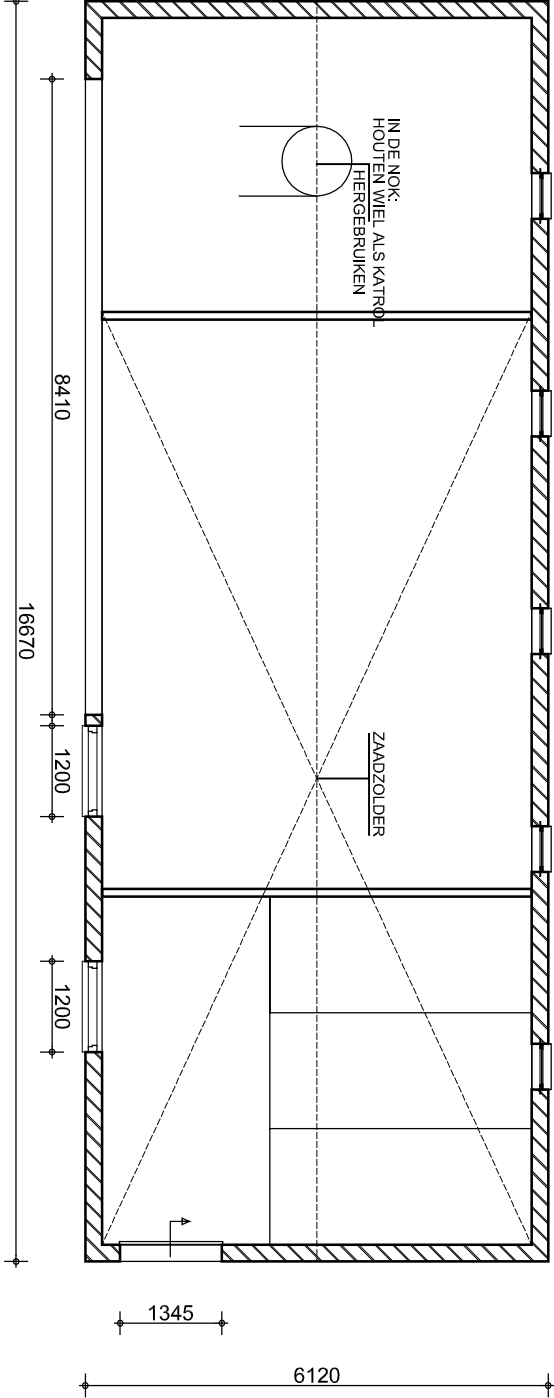
PLATTEGROND BEGANEGROND
