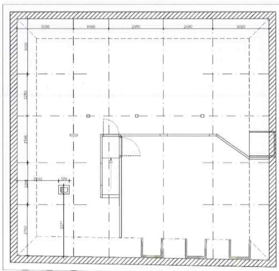
PLATTEGROND VERDIEPING
