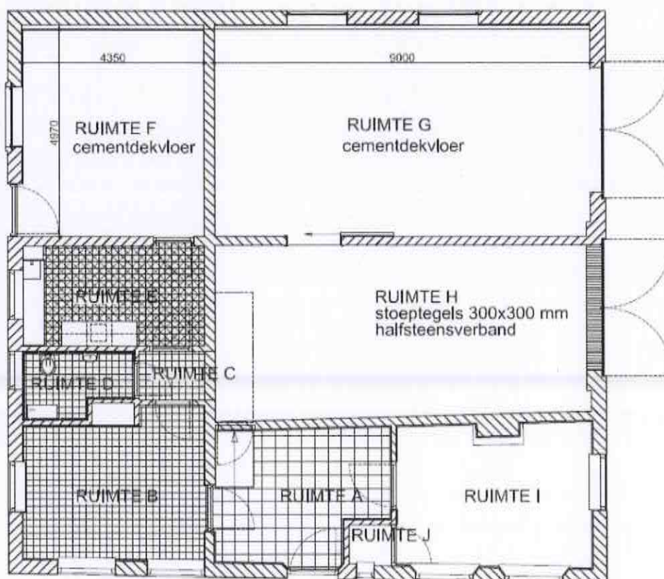
PLATTEGROND BEGANEGROND
