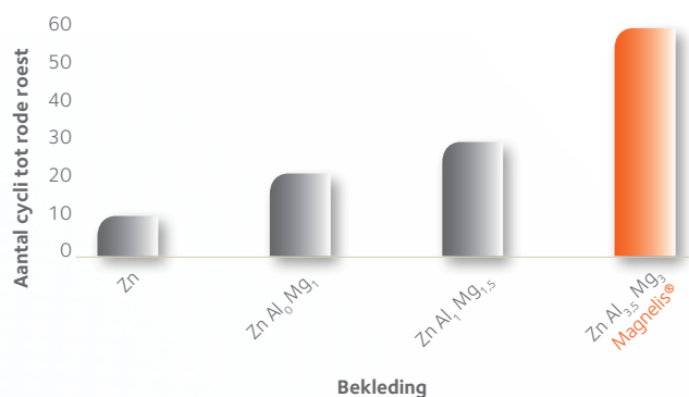
Corrosieweerstand van bekledingen met verschillende Zn-, Al- en Mg-samenstellingen in een cyclische test
