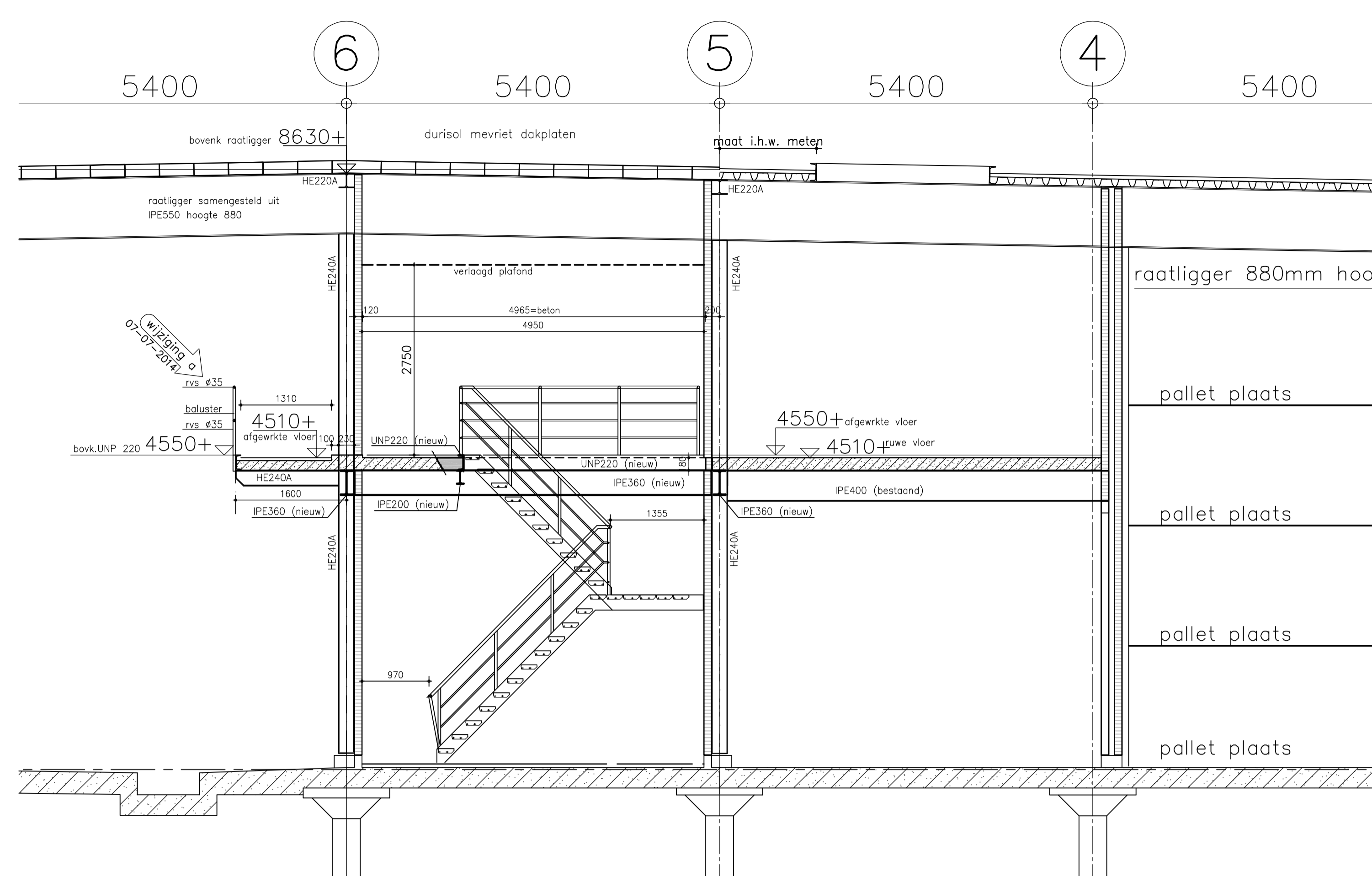
doorsnede B-B
