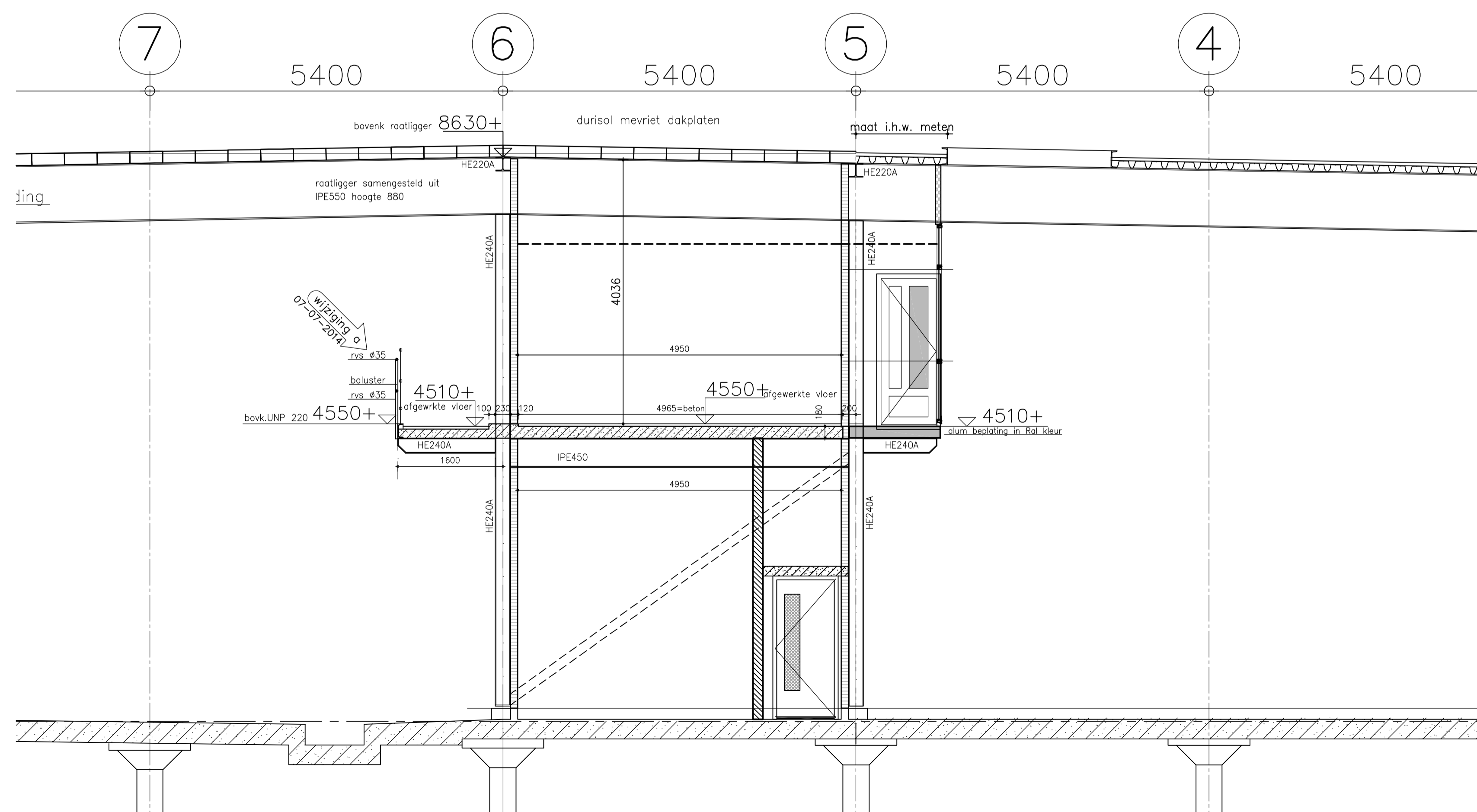
doorsnede C-C
