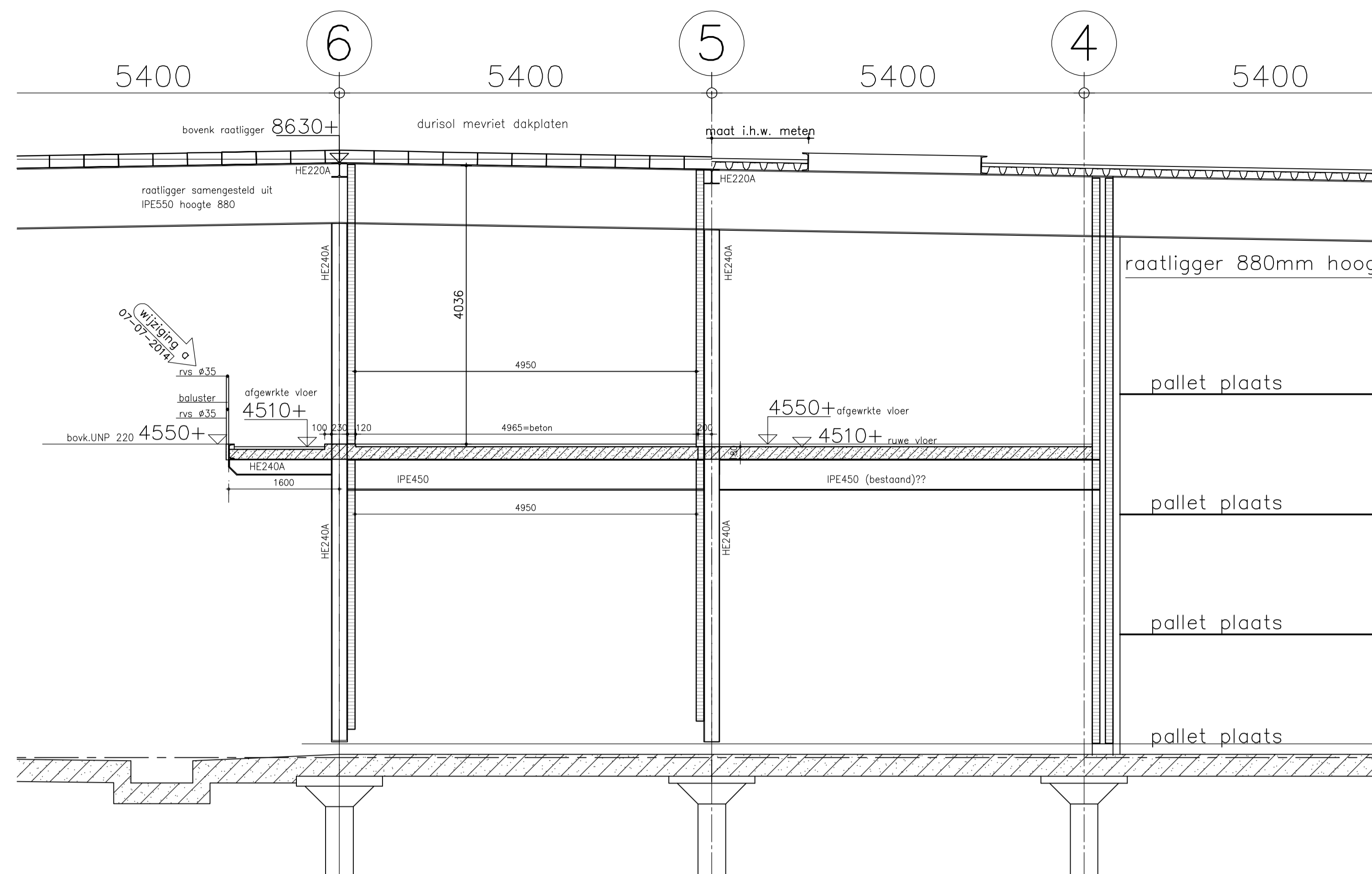
doorsnede A-A
