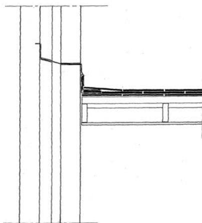
Detail 9d. Aansluiting aan opgaand metselwerk
