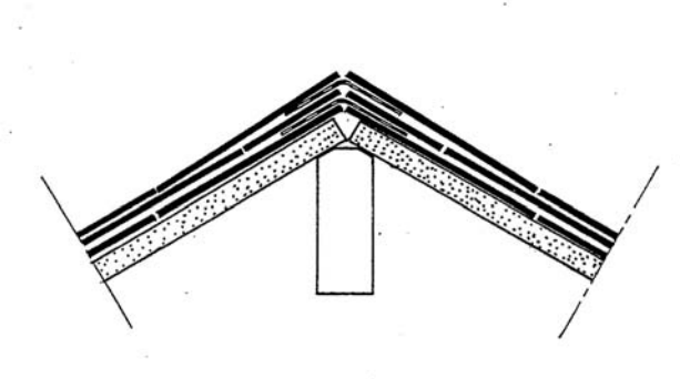
Detail 6a. Hoekkeperaansluiting
