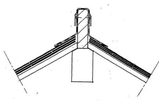
Detail 6b. Hoekkeperaansluiting
