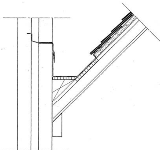
Detail 10c. Boven aansluiting schoorsteen
