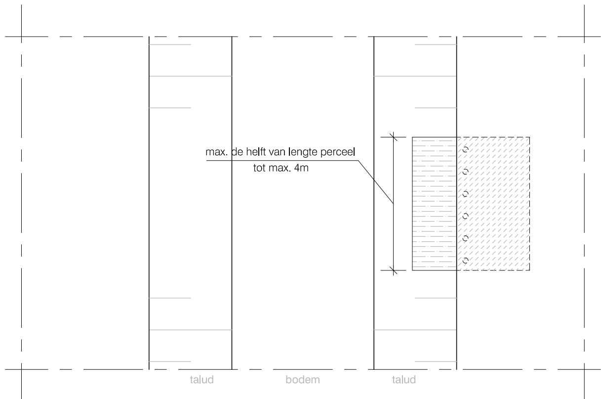
Bovenaanzicht
