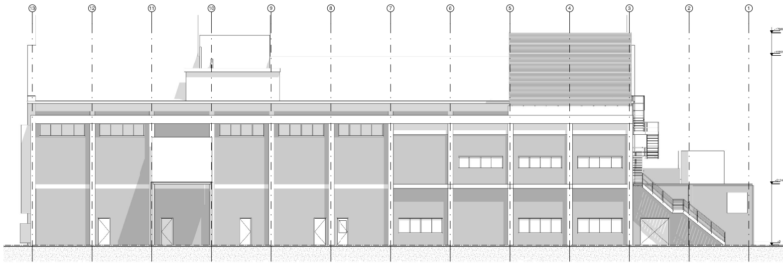
rechtergevel
