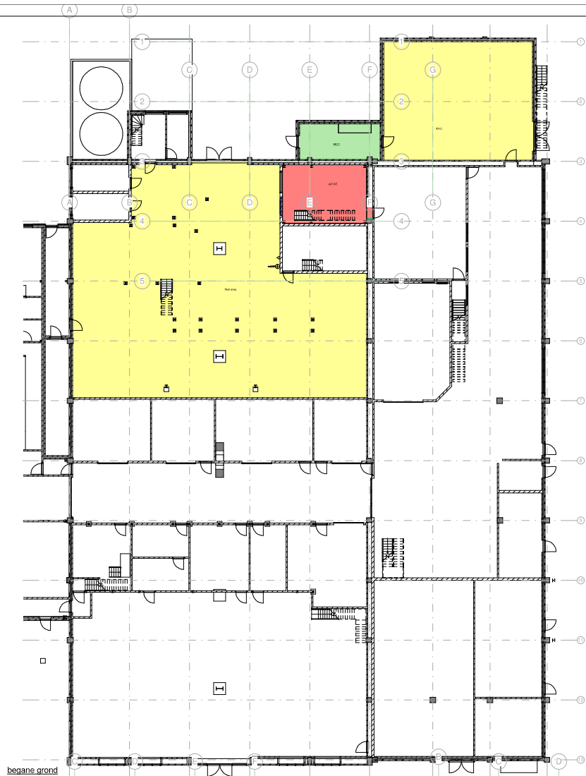
begane grond
