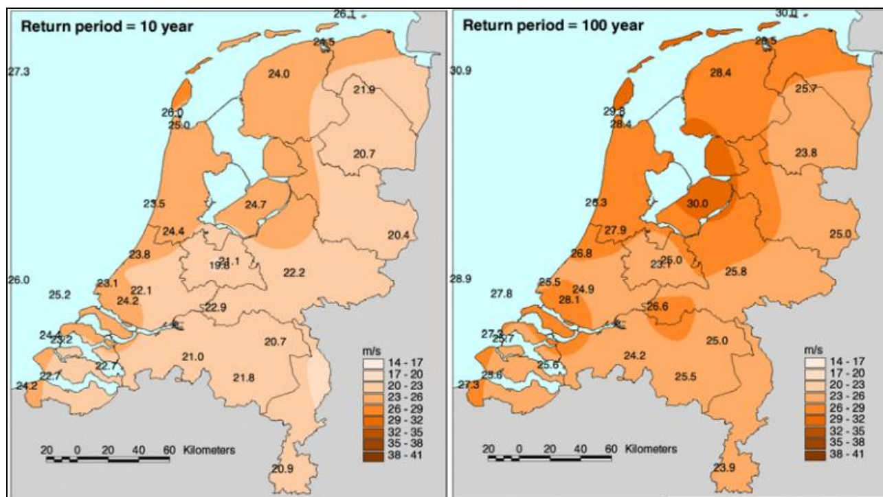
Figuur 1 : Windsnelheid in Nederland met een herhalingsijd van 10 en 100 jaar
