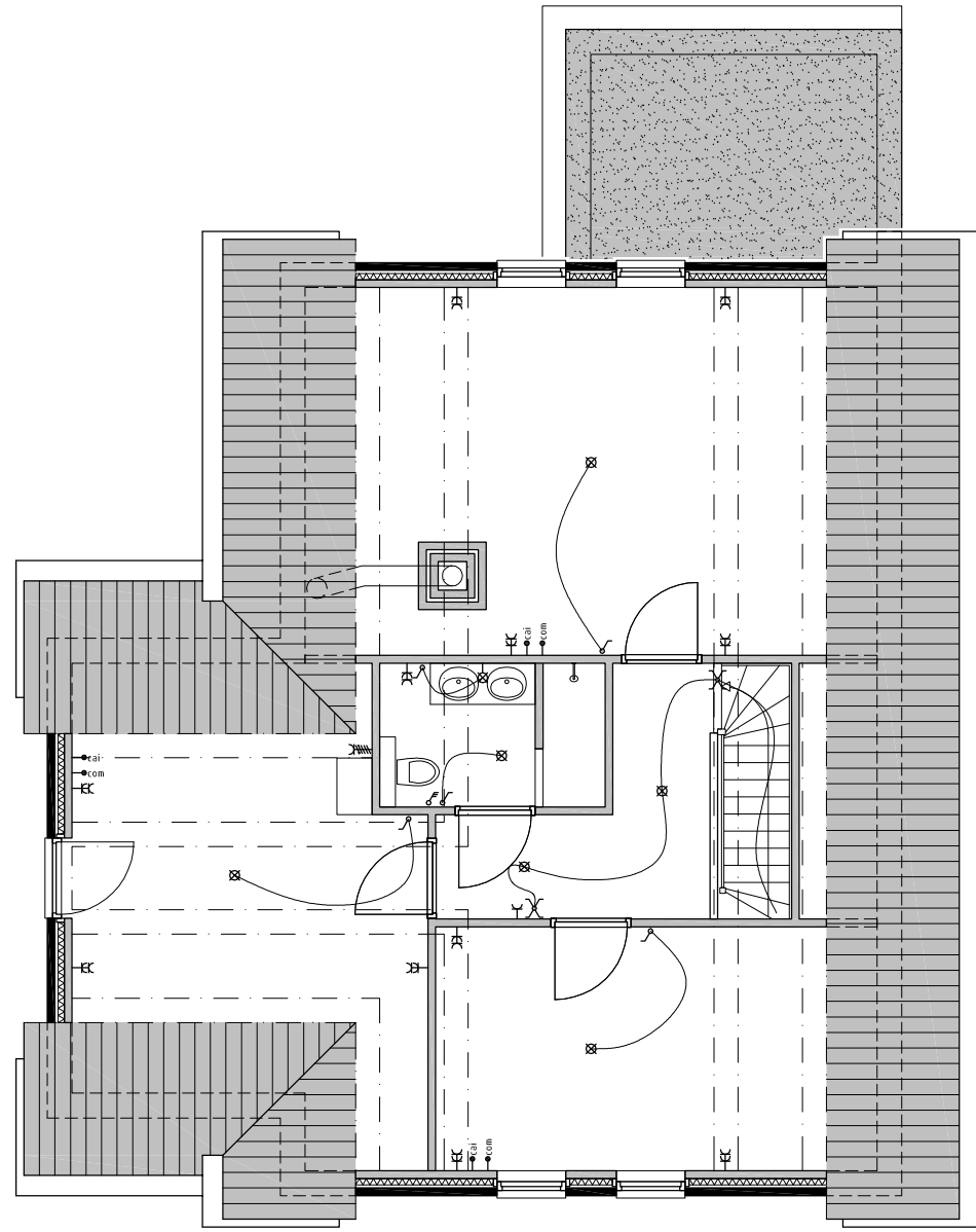
Elektrische installatie principe Verdieping
