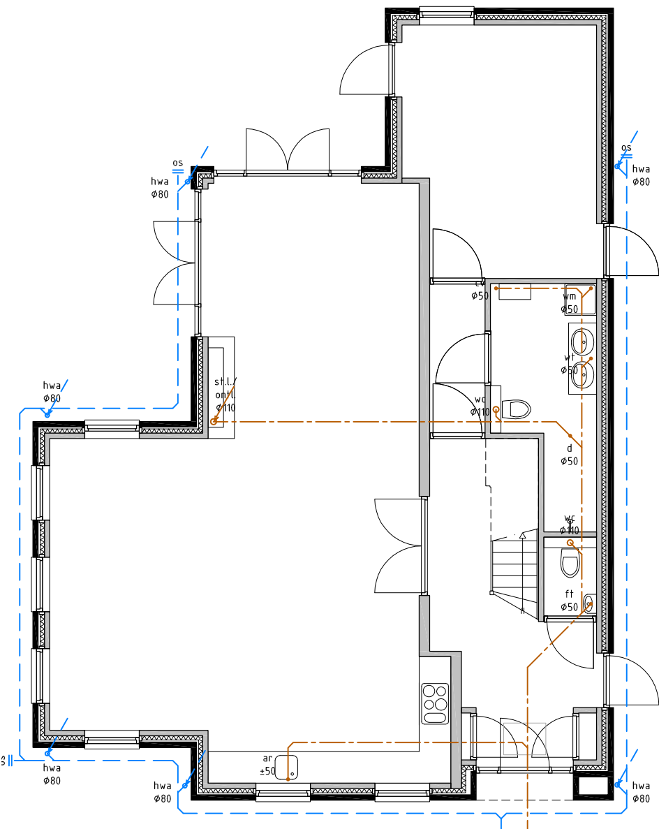
Rioleringsinstallatie principe Begane grond
