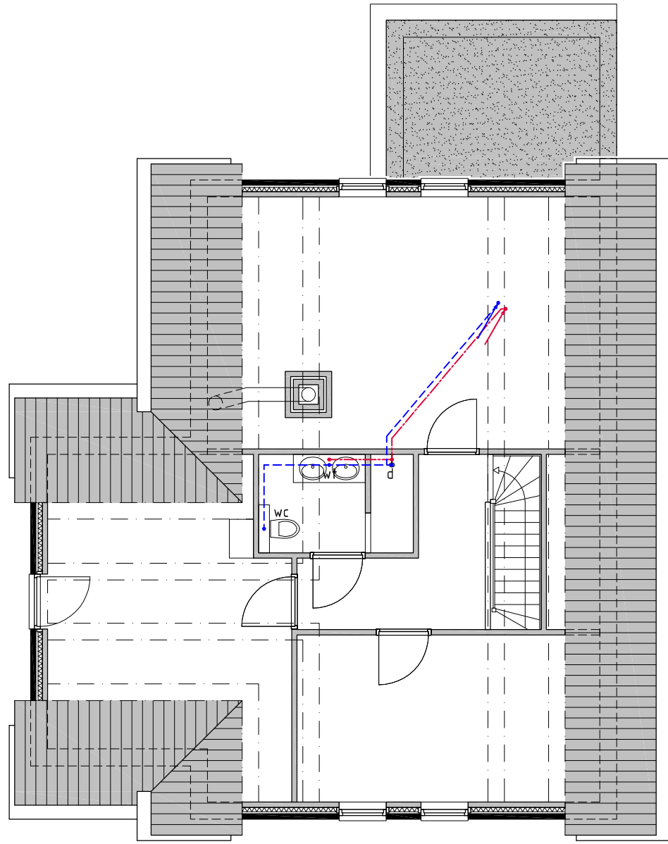
Waterinstallatie principe Verdieping
