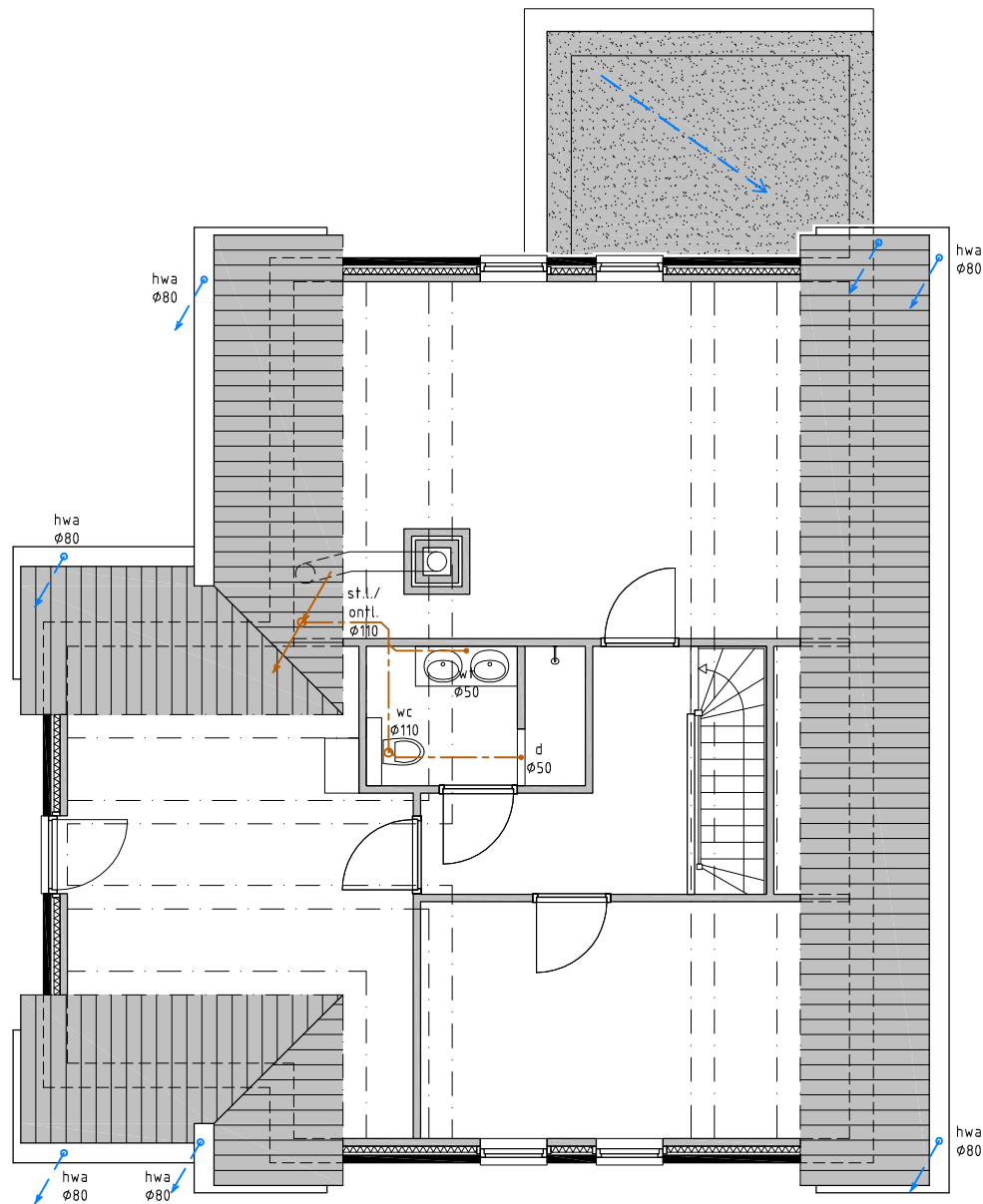
Rioleringsinstallatie principe Verdieping
