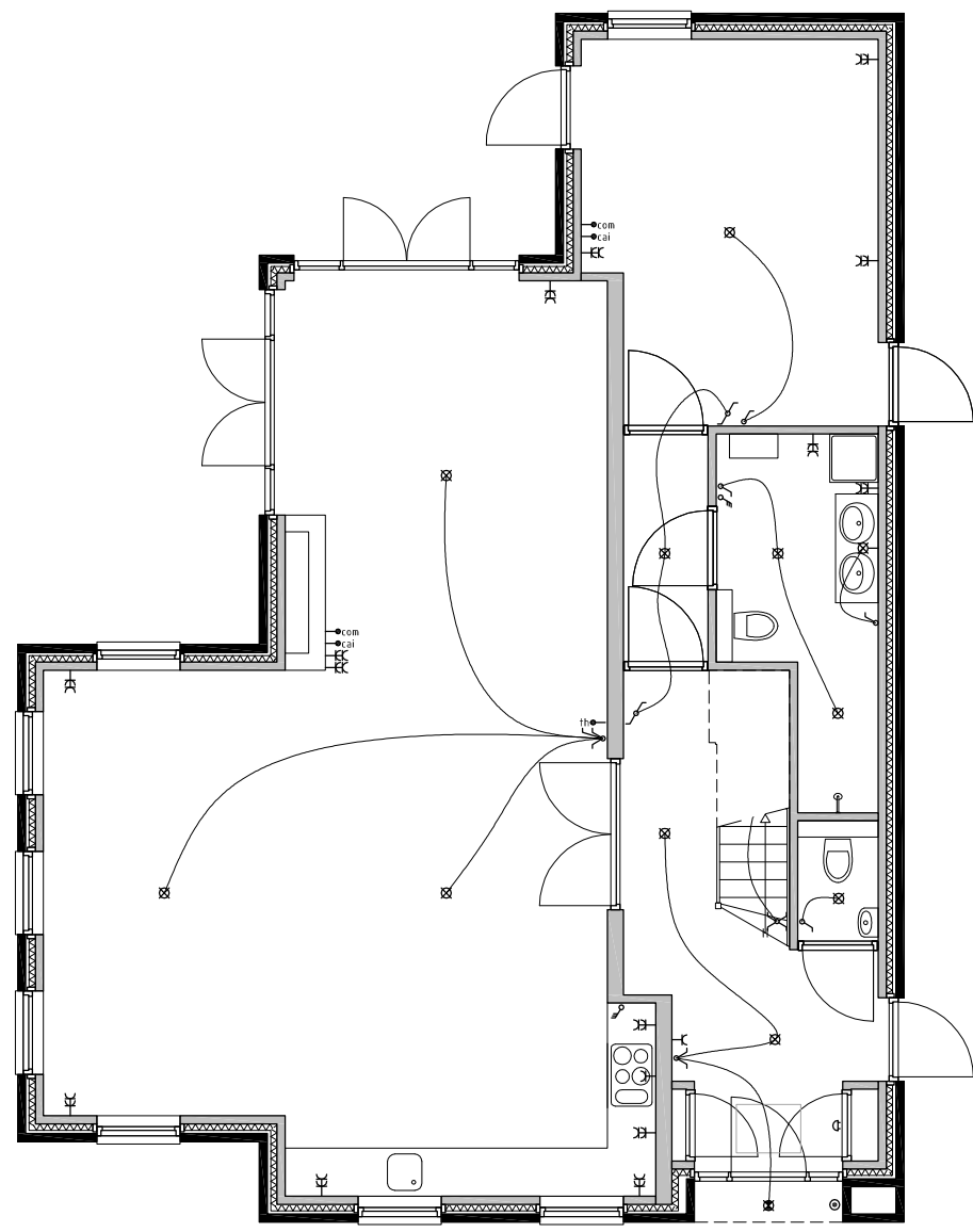
Elektrische installatie principe Begane grond
