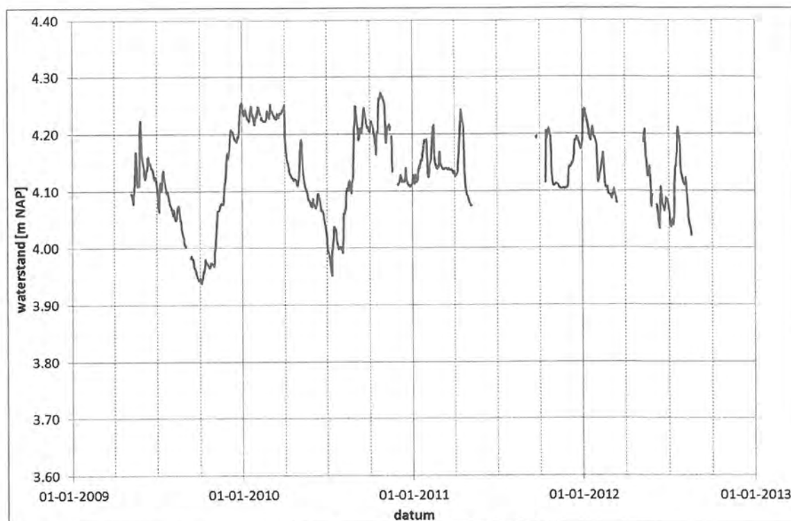
Figuur 18 Metingen oppervlaktewaterstand vijver Brederode 2009-2012
