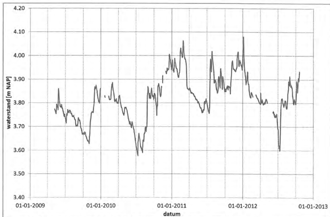
Figuur 17 Metingen oppervlaktewaterstand vijverpartij Halve Maantje 2009-2012
