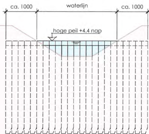
vooraanzicht te plaatsen stuw
