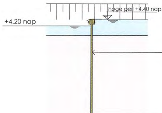
doorsnede te plaatsen stuw
