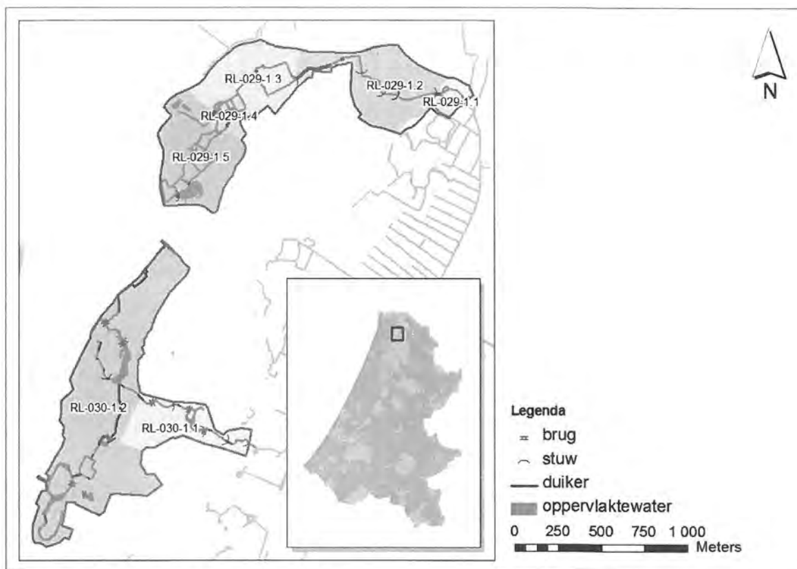
Figuur 11 Watersysteem en peilvakindeling
