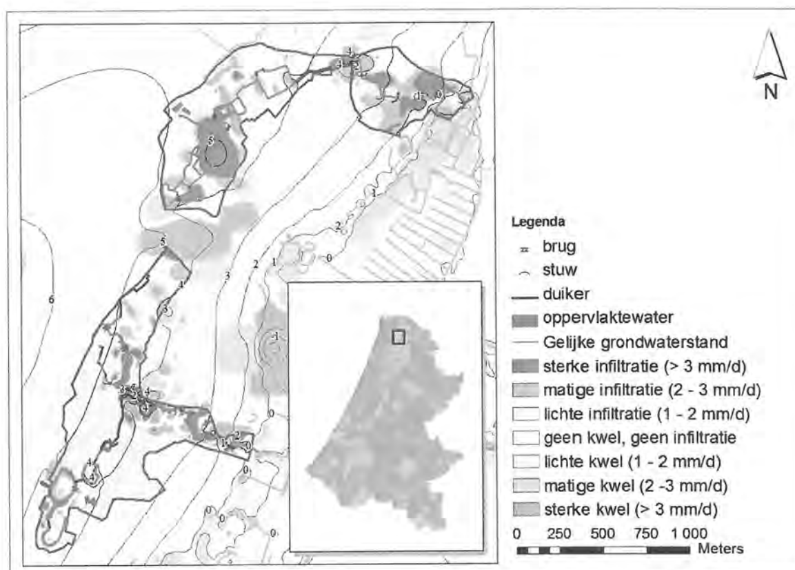
Figuur 10 Grondwaterstand, kwel en infiltratie
