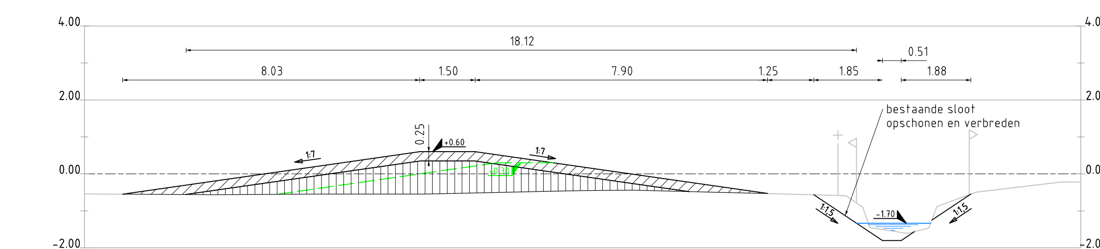
Dwarsprofiel B1
