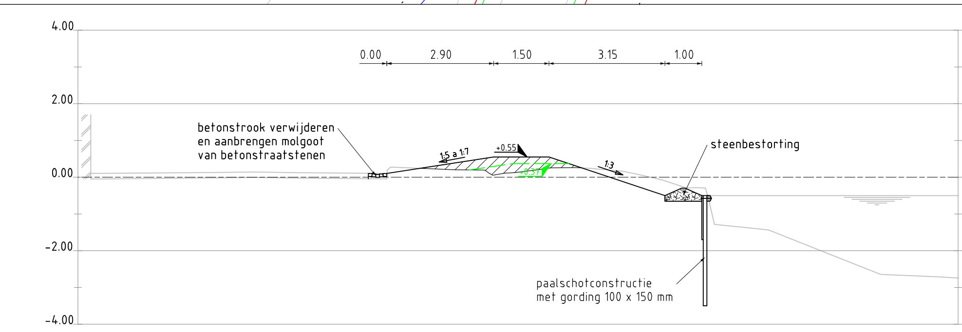
Dwarsprofiel A4
