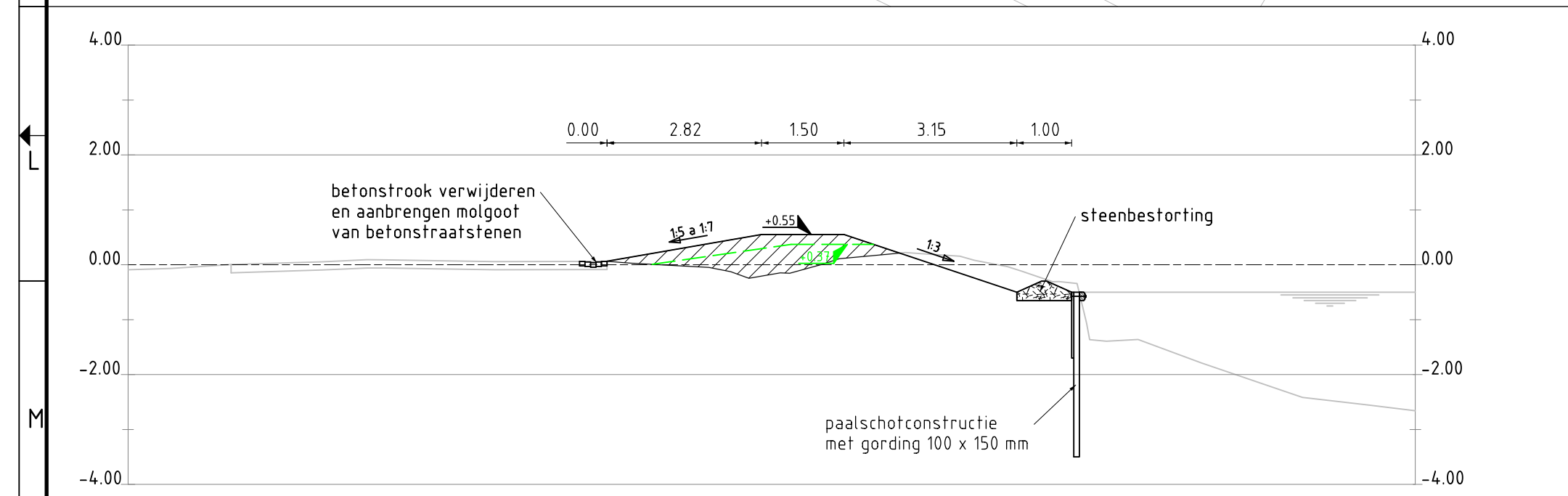
Dwarsprofiel A3
