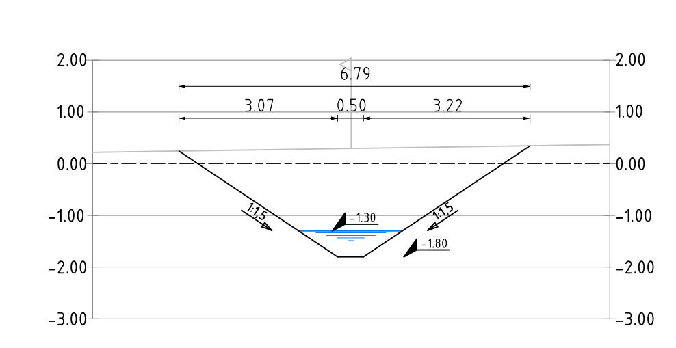
Dwarsprofiel A9
