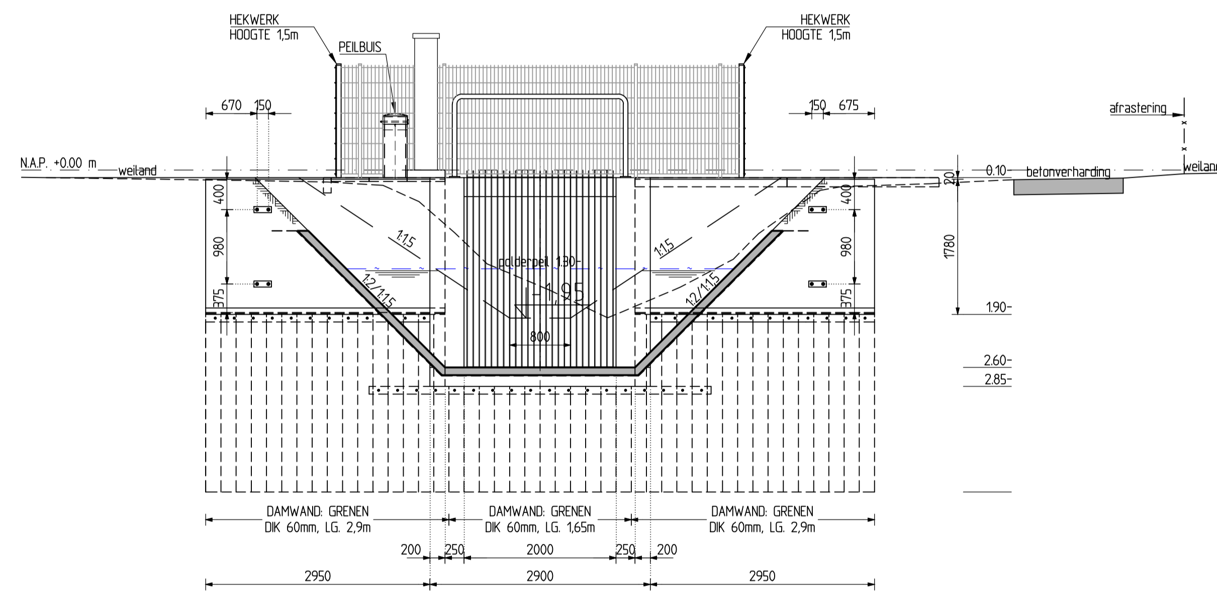
AANZICHT INSTROOMZIJD SCHAAL 150
