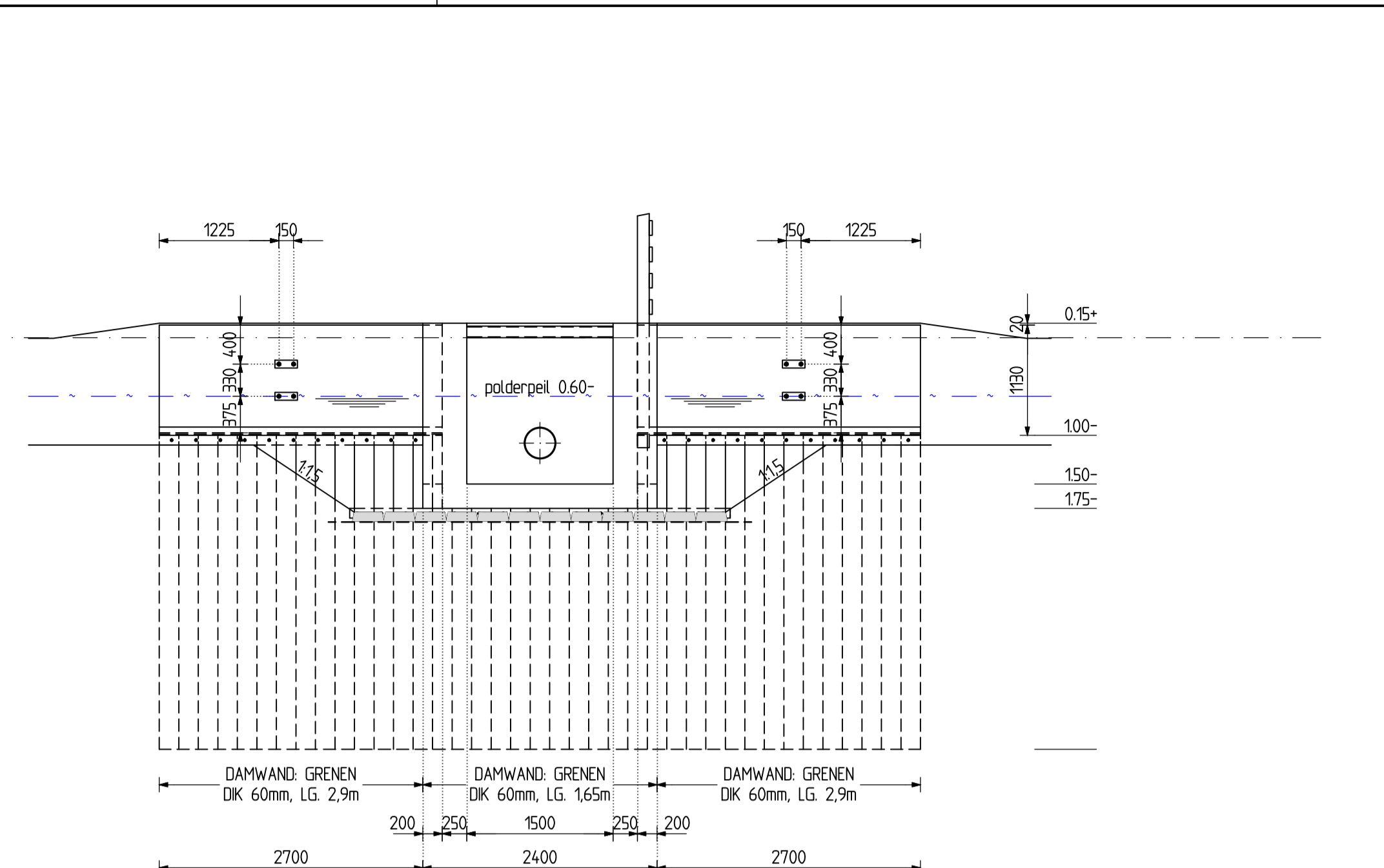
AANZICHT UITSTROOMZIJD SCHAAL 150
