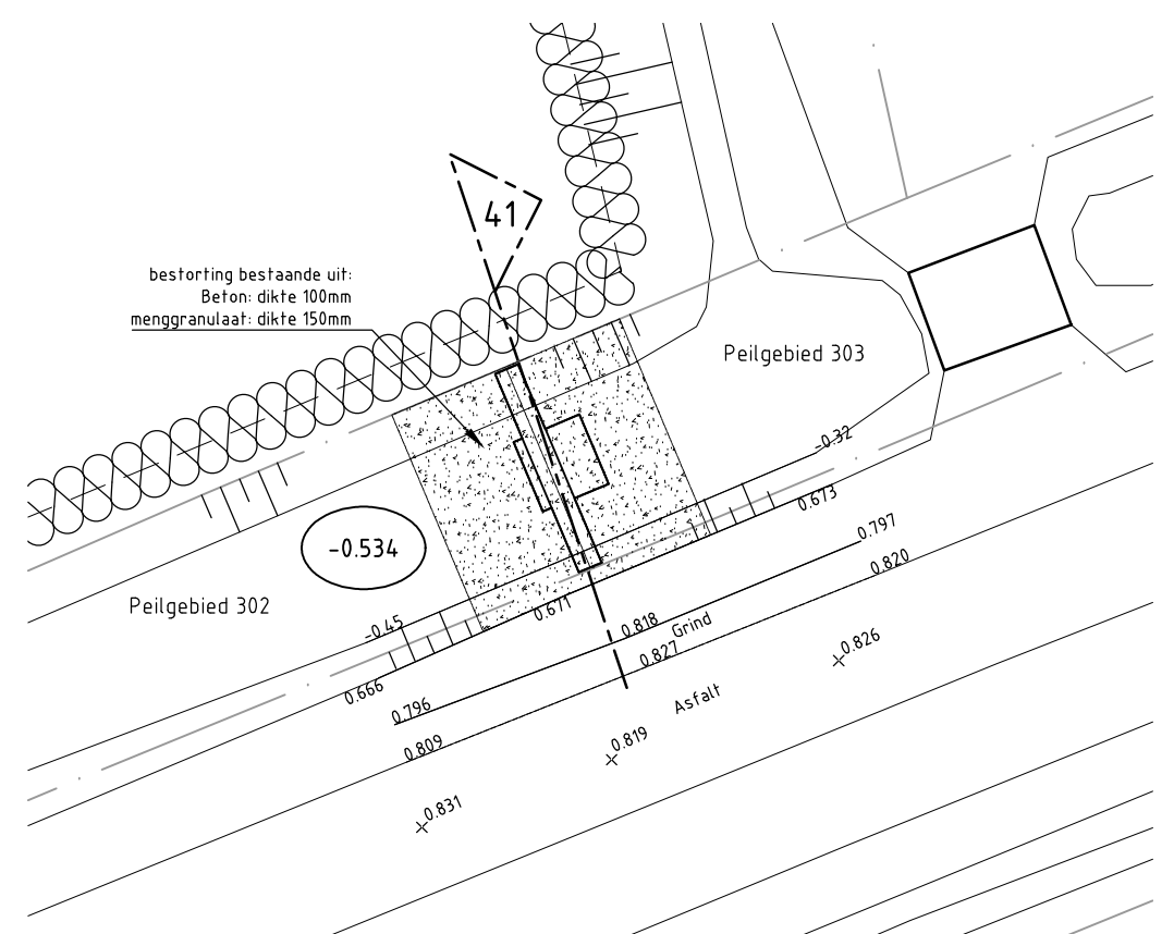
Situatie stuw schaal1:200
