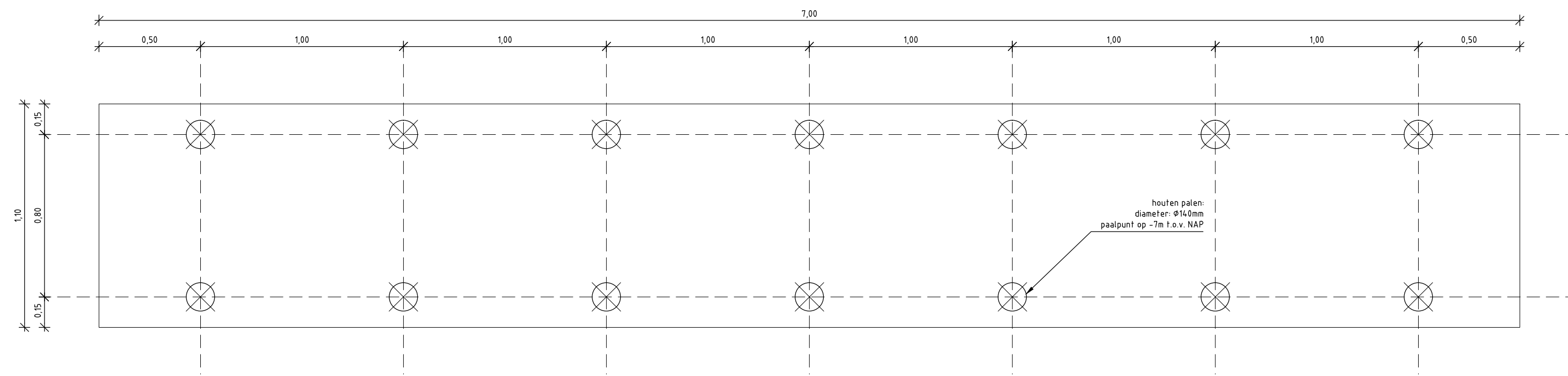
Palenplan schaal1:20
