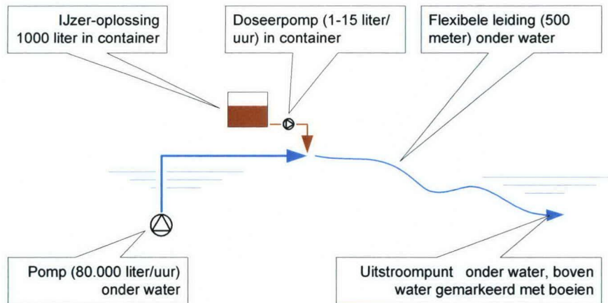
Figuur 1: Principe ijzerdosering Sloene
