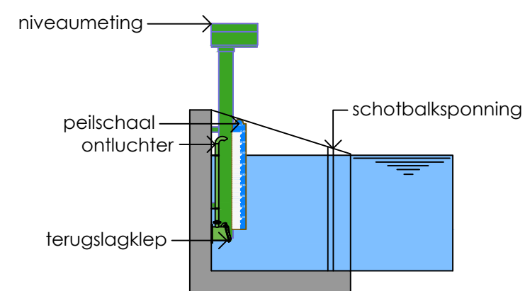
Doorsnede B-B 1:50
