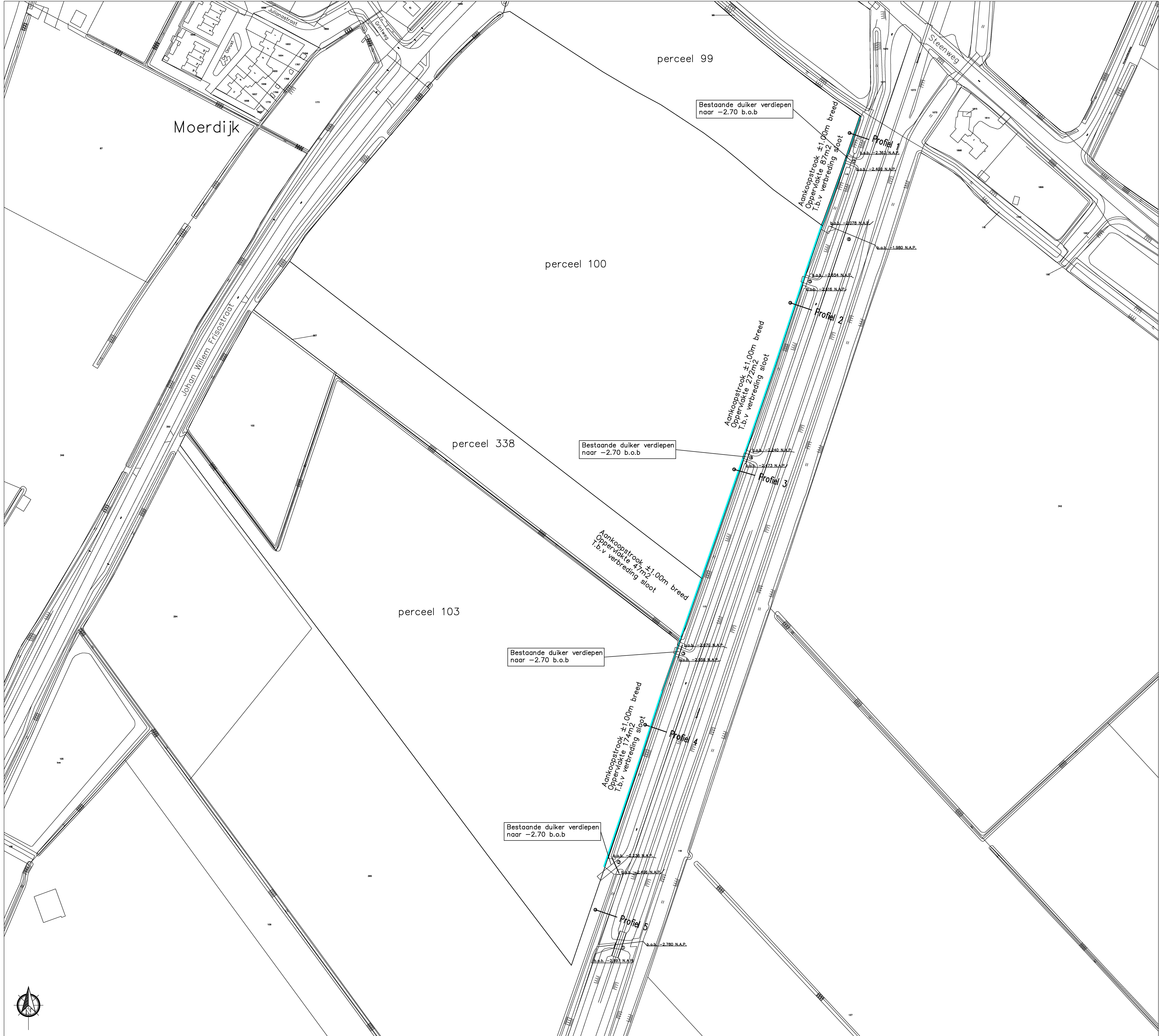
Overzichtstekening schaal 1:1000
