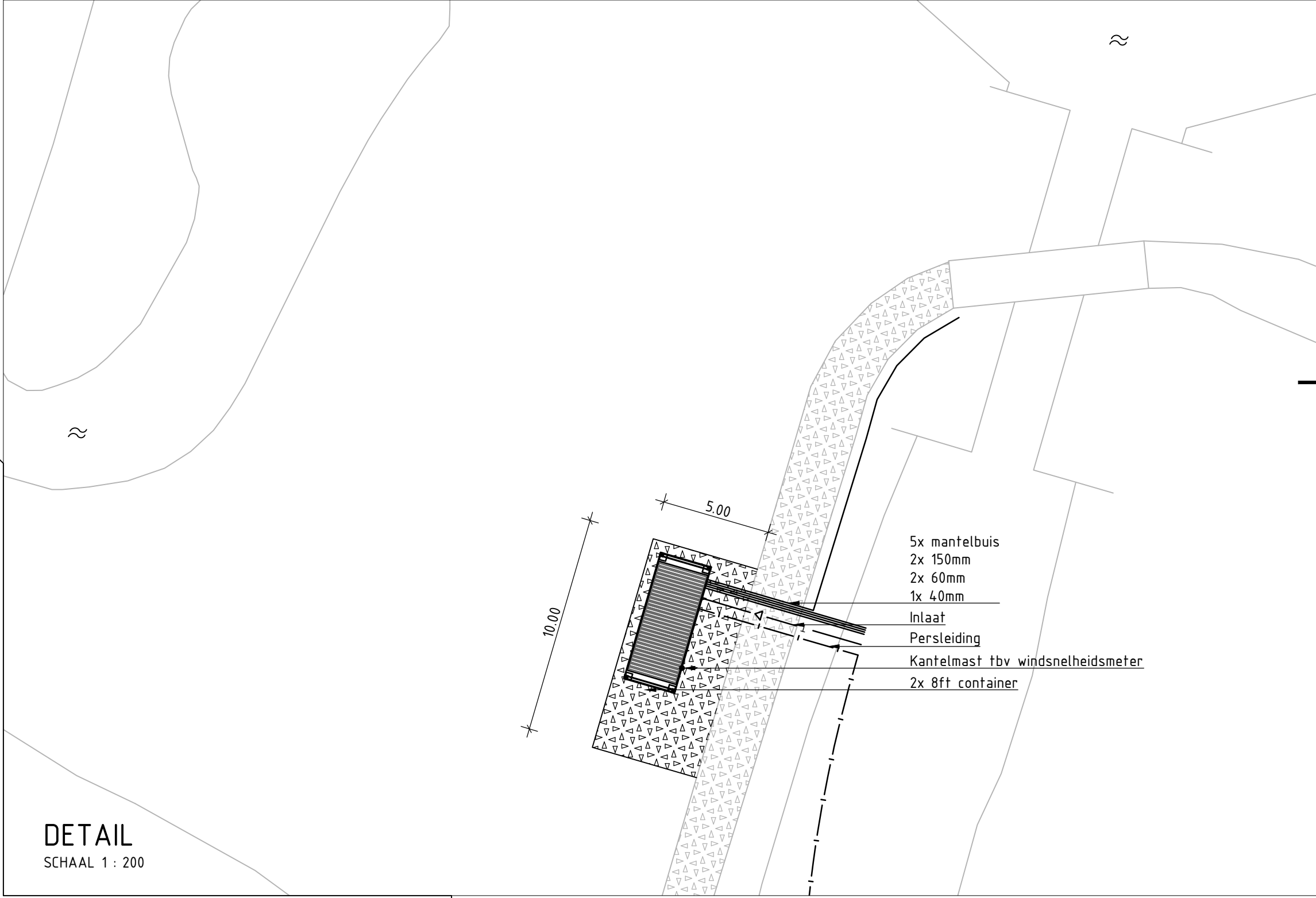
DETAIL INHOUD CONTAINER SCHAAL 1 : 20
