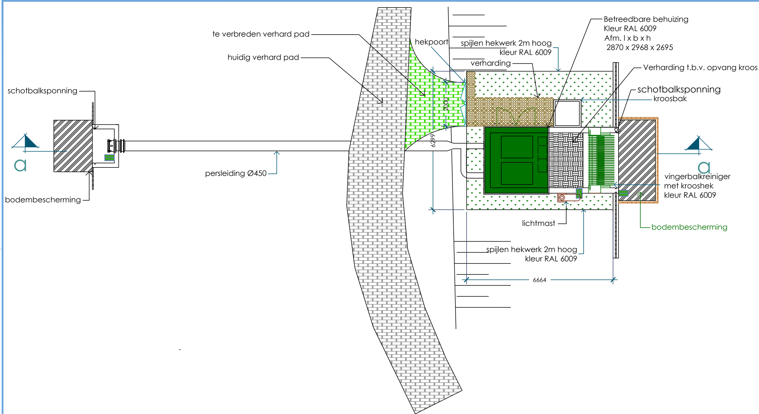
bovenaanzicht 1:100
