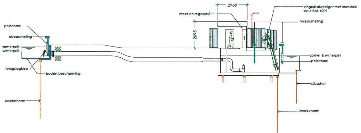
Figuur 3B Langsdoorsnede
