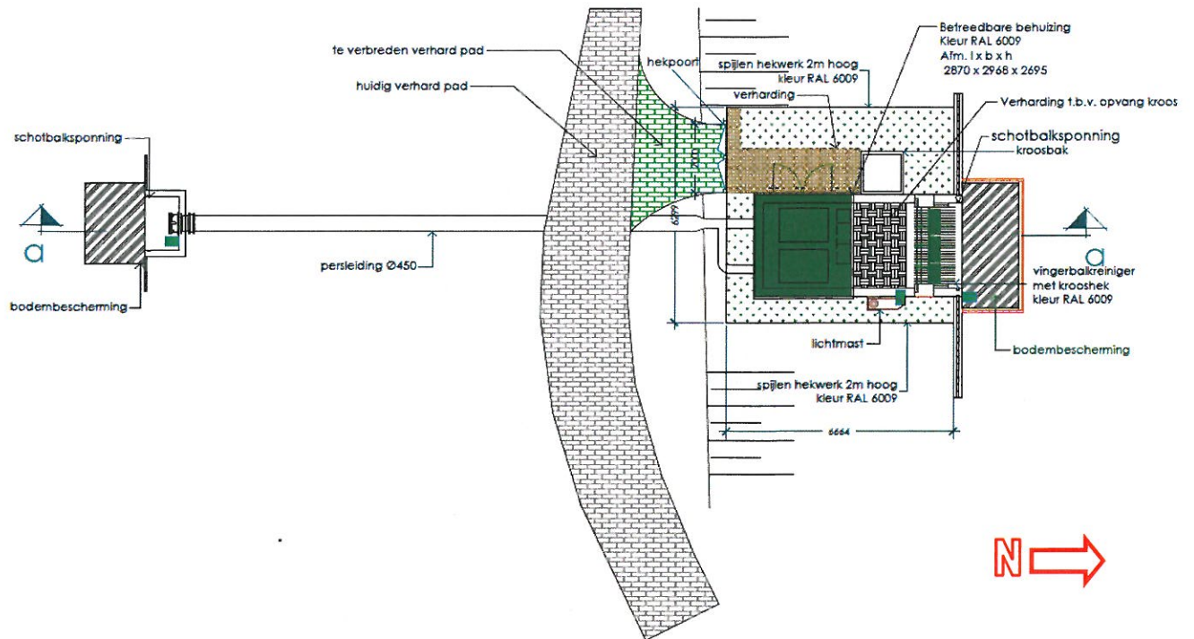
Figuur 3A Bovenaanzicht
