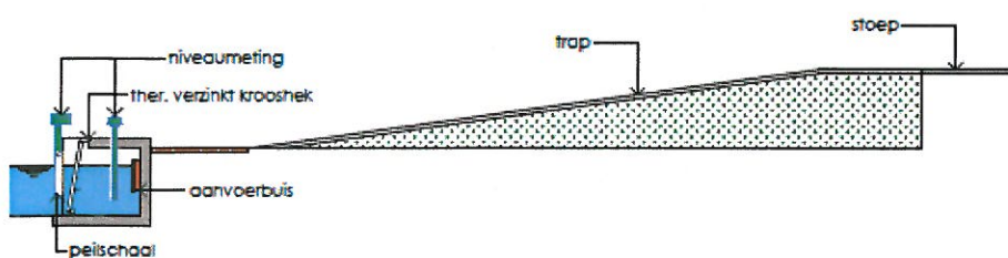
Figuur 3B Langsdoorsnede
