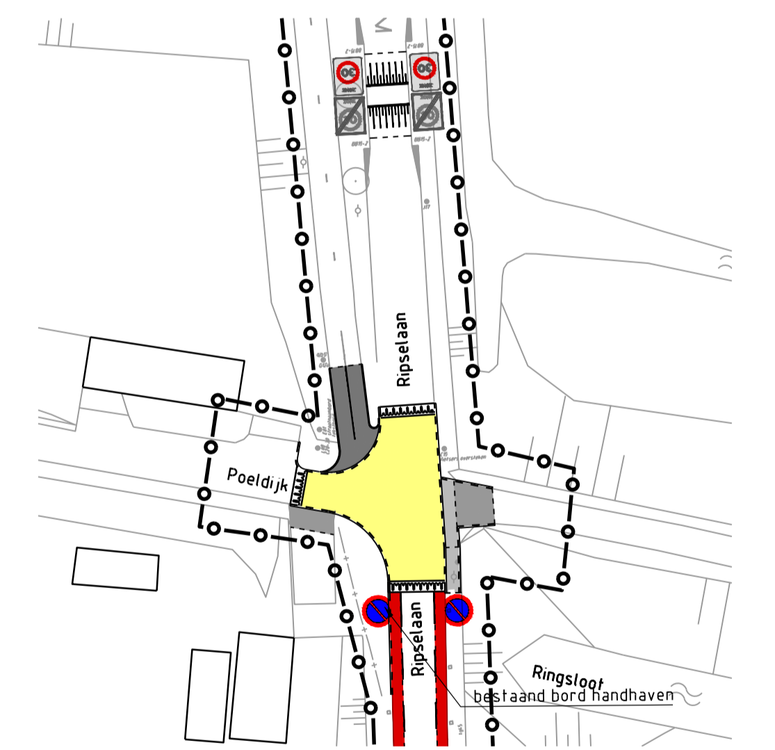
Inrichting kruising
