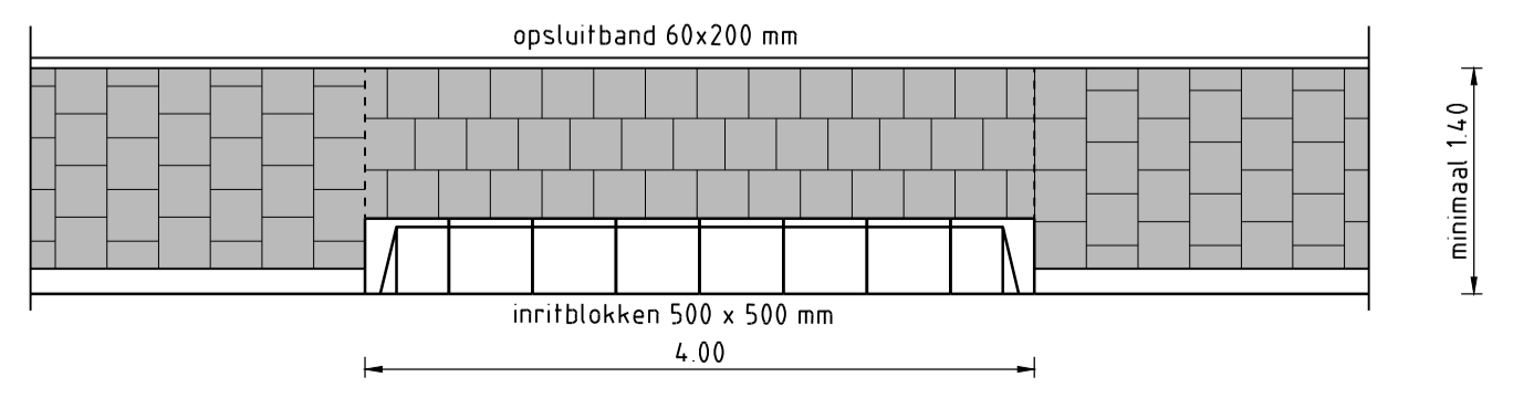
Principe profiel inrit Koppoellaan
