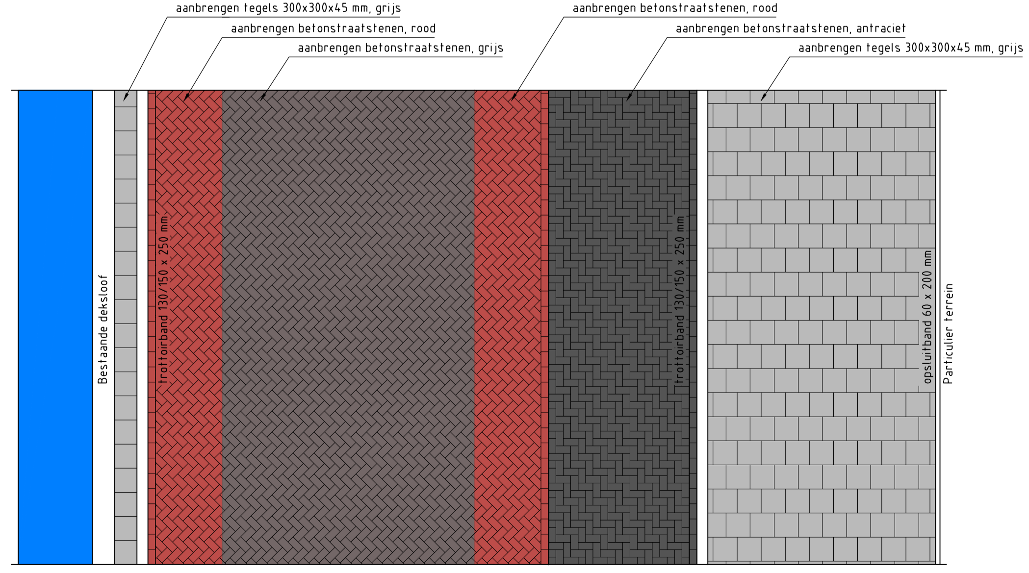
Principe profiel Koppoellaan
