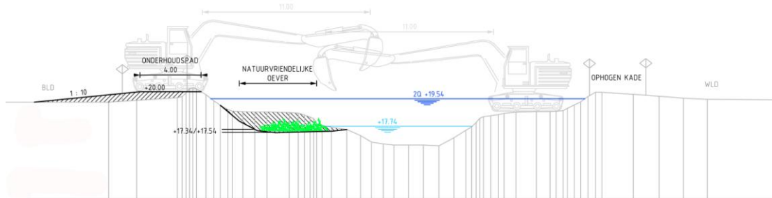
Figuur 1: principe profiel natuurvriendelijke inrichting oever Buurserbeek
