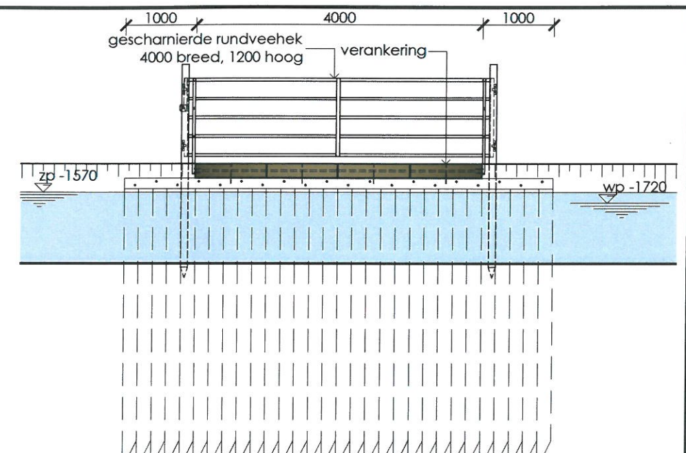
doorsnede b-b 1:50
