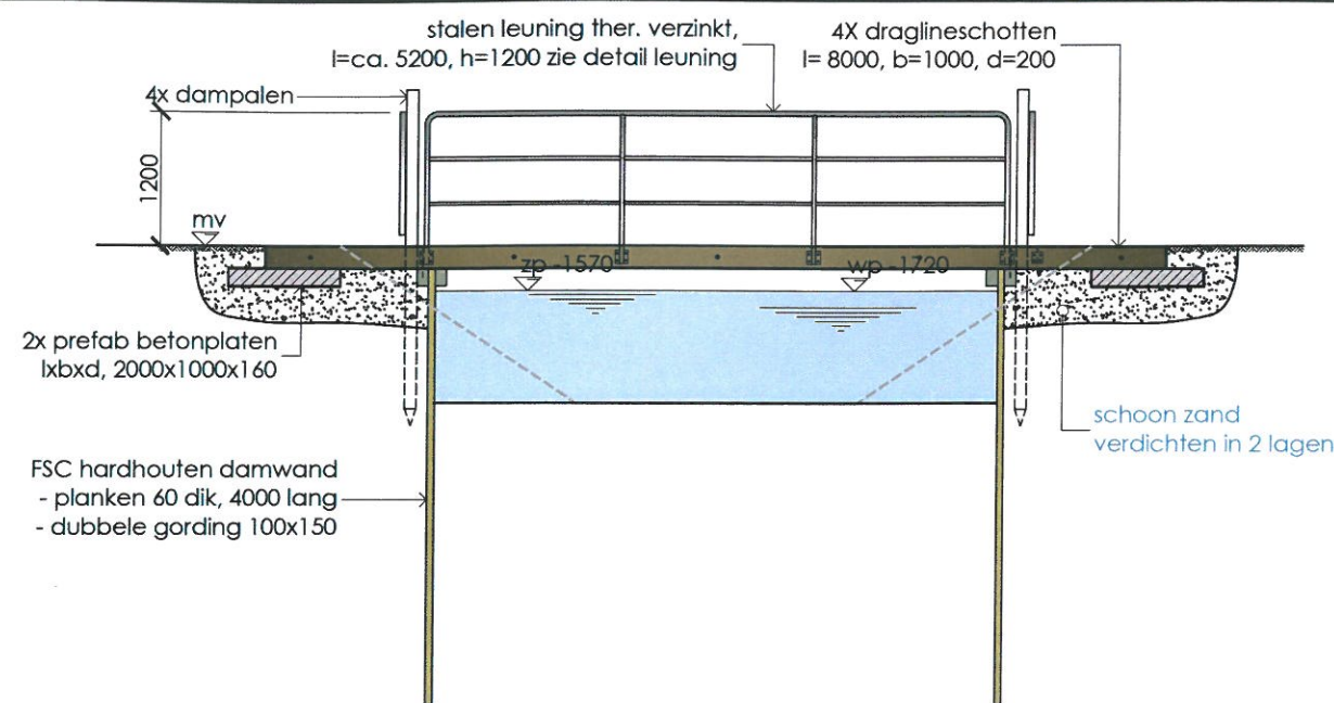
doorsnede a-a 1:50
