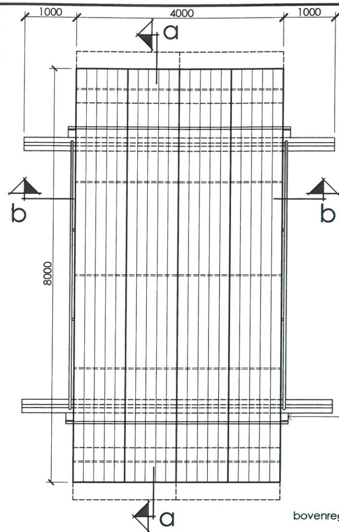
bovenaanzicht 1:50
