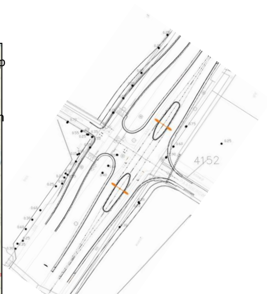
Locatie halte Paasbergweg aan de N342 Oldenzaal – Denekamp en voorlopig ontwerp met middengeleiders
