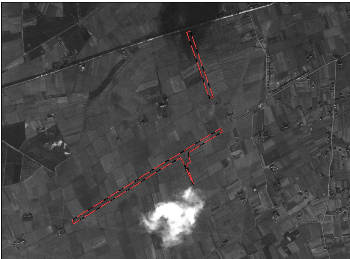
Figuur 3: Overzicht van de luchtfotodekking voor het project "Ecologische verbindingzone Zwarte Sloop".
