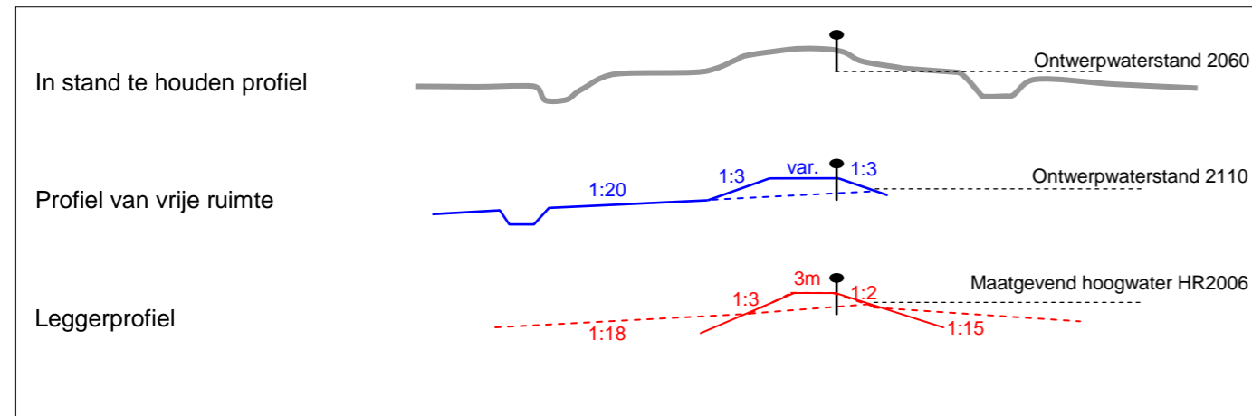
Figuur 2: Maatvoering profielen
