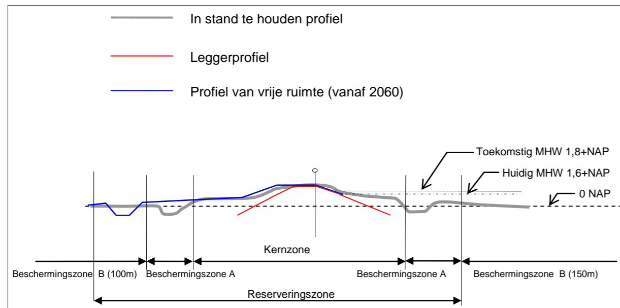
Figuur 1: schematische weergave van profielen en zones
