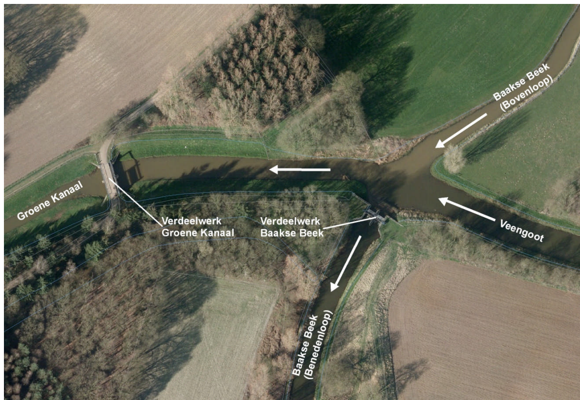
Figuur 1: Verdeelwerk Baakse Beek en Groene Kanaal
