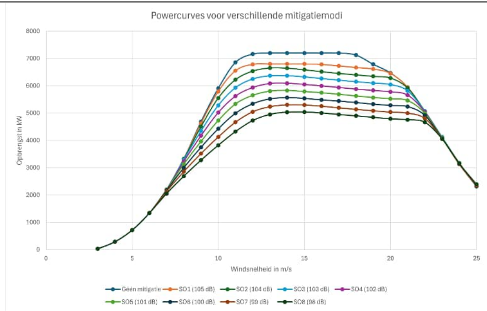
Figuur 18 Powercurves van de Vestas V172-7.2MW, zowel zonder mitigatie, als voor de verschillende mitigatiemodi.
