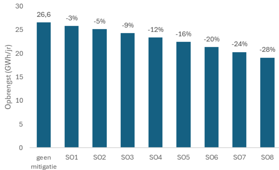
Figuur 20 De gemiddelde jaaropbrengst voor de verschillende mitigatiemodi uit Figuur 18, indien de windturbine continu in een bepaalde modus zou draaien.
