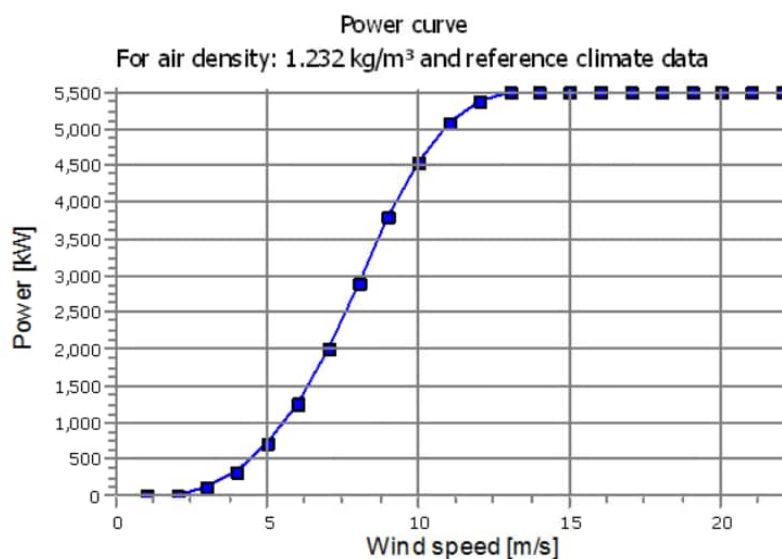
Afbeelding 7.5 Power curve van de ondergrens windturbine (Enercon E160)
