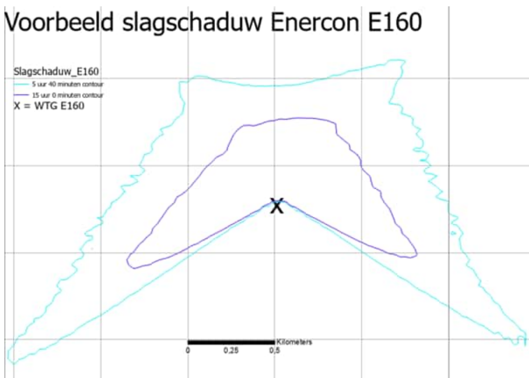
Afbeelding 7.2 Slagschaduw contouren van voorbeeld windturbine (Enercon E160)
