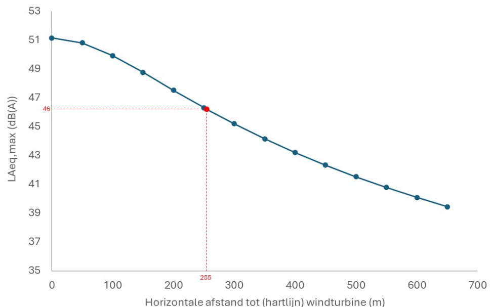
Figuur 27 Verhouding tussen L_{Aeq} en afstand tot windturbine
