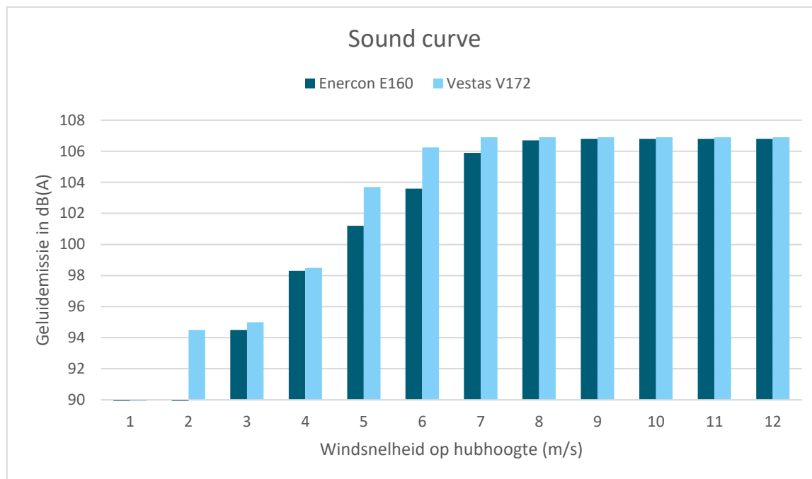
Afbeelding 7.1 Sound curve van de turbines
