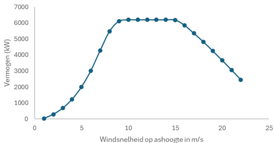
Figuur 23 Powercurve van de Vestas V162-6.2MW, de ondergrens van de bandbreedte van het VKA.
