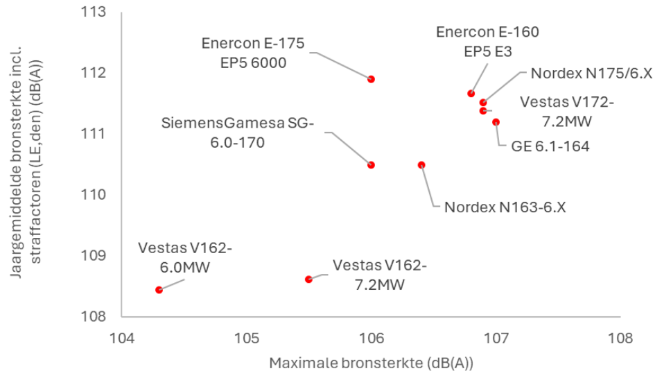
Figuur 26 Illustratie van de stelling dat een hogere maximale bronsterkte (horizontale as) niet per se leidt tot een hogere jaargemiddelde bronsterkte (verticale as).
