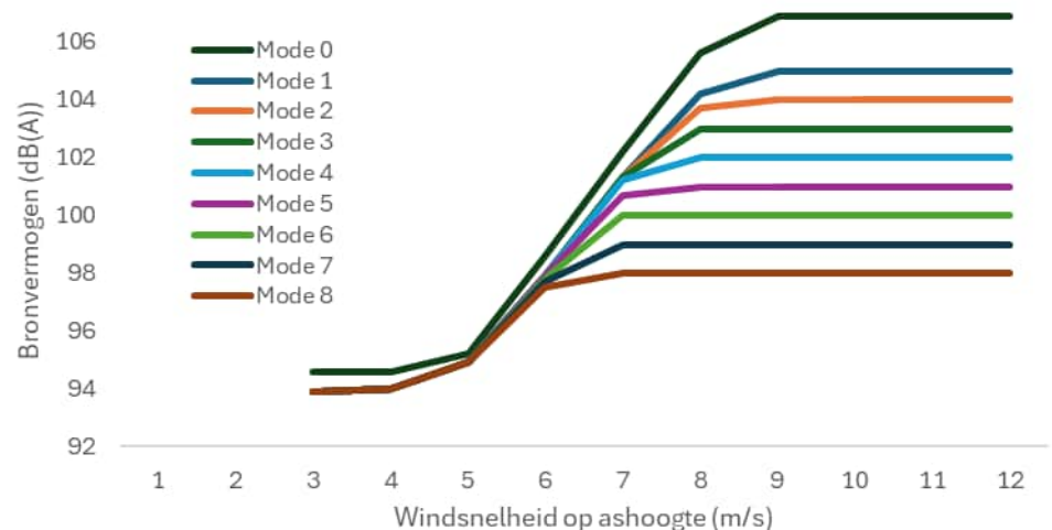
Figuur 19 Geluidscures van de Vestas V172-7.2MW, zowel zonder mitigatie (Mode 0), als voor de verschillende mitigatiemodi. De powercurves uit Figuur 18 corresponderen met deze geluidscures.
