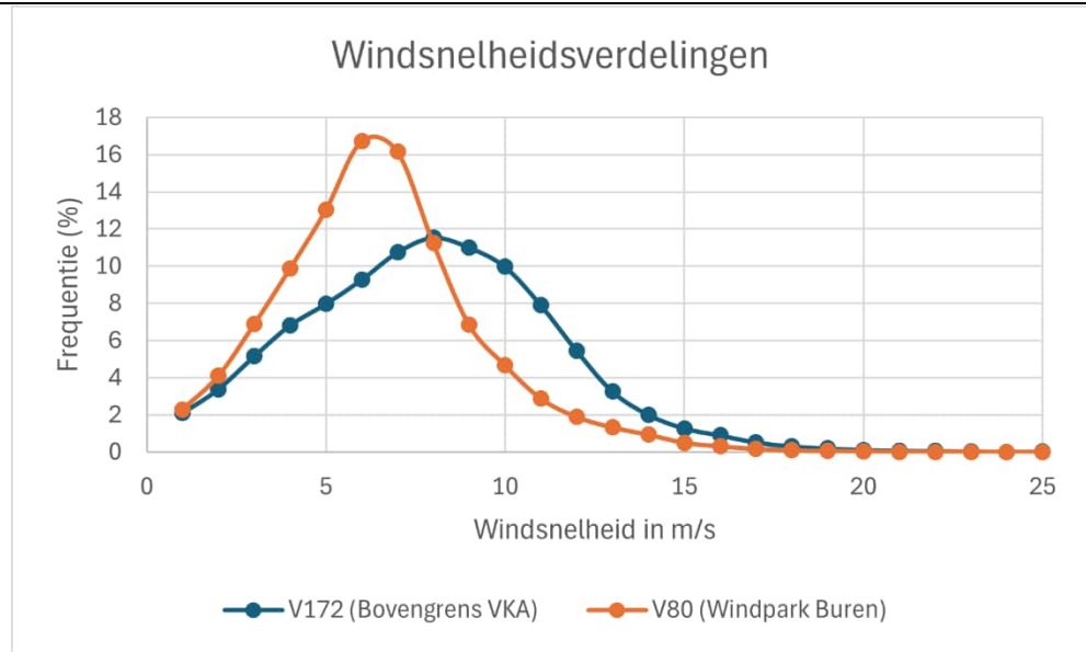
Figuur 17 Percentage van de tijd (etmaalgemiddeld) dat de wind in een bepaalde windklasse waait.
