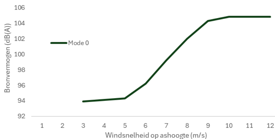
Figuur 24 Geluidscurve van de Vestas V162-6.2MW zonder mitigatie (Mode 0). De powercurve uit Figuur 23 correspondeert met deze geluidscures.
