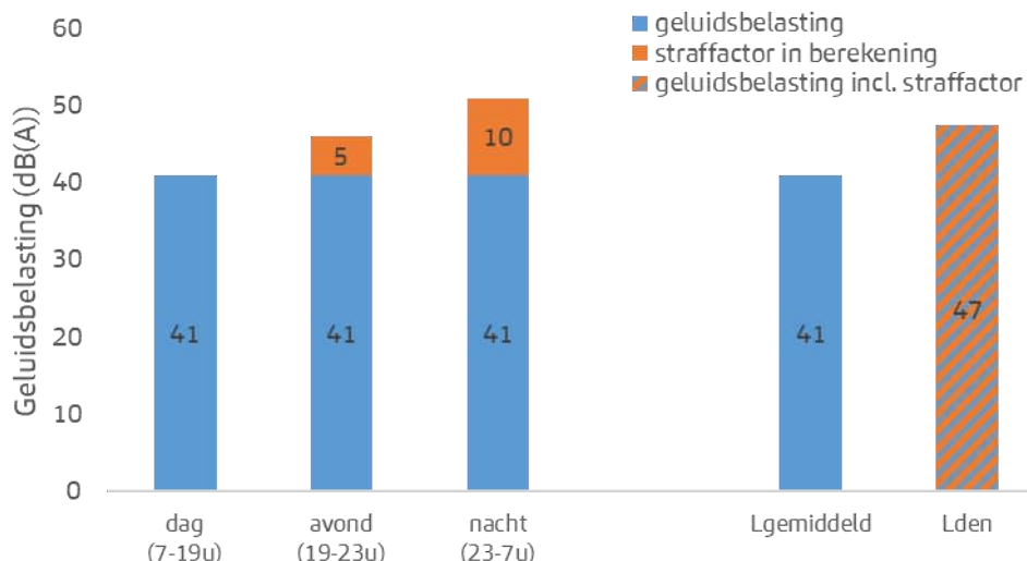
Figuur 13 Grafische weergave L_{den} . Dit voorbeeld is een denkbeeldige situatie waarin een geluidsbron een continue belasting van 41 dB(A) op een toetspunt veroorzaakt.
