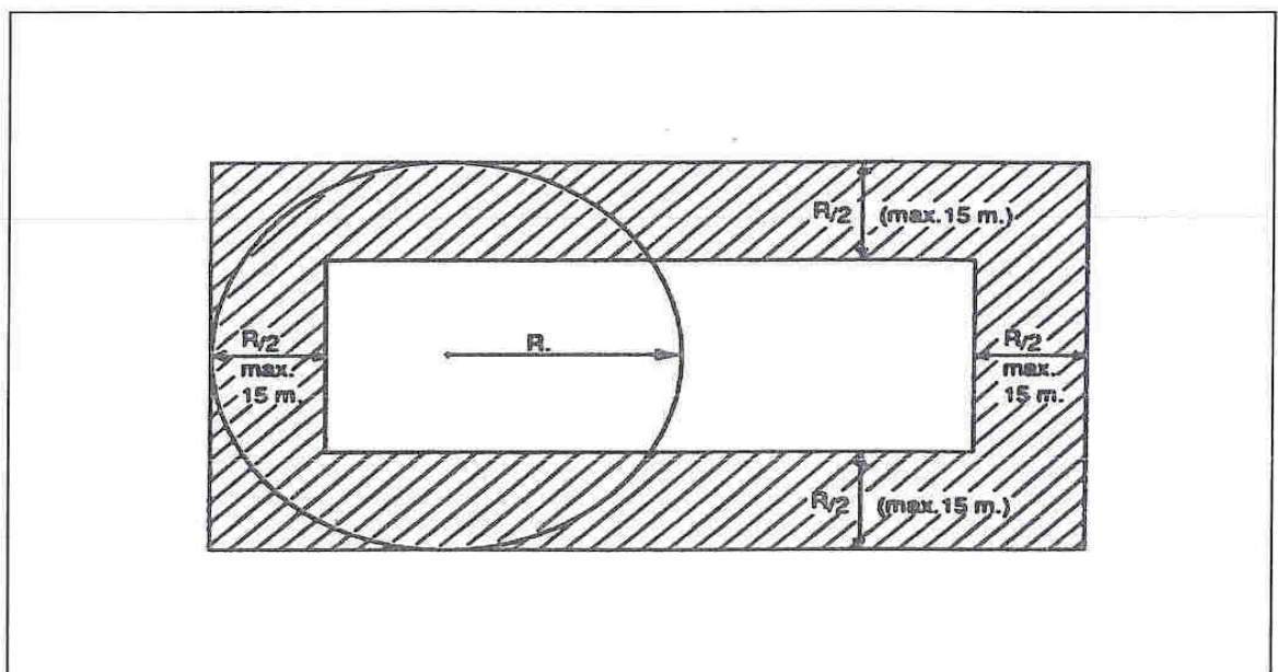
Figuur 2 Voor verkeer vrij te houden hoogten (artikelen 2.5.7 en 2.5.8)
