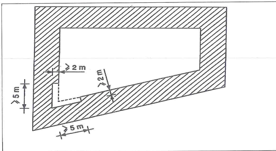
Figuur 11 Teruglegging met het oog op de daglicht toetreding van achtergevelrooilijn die een scherpe hoek met elkaar vormen (ingevolge artikel 2.5.11, lid 2)
