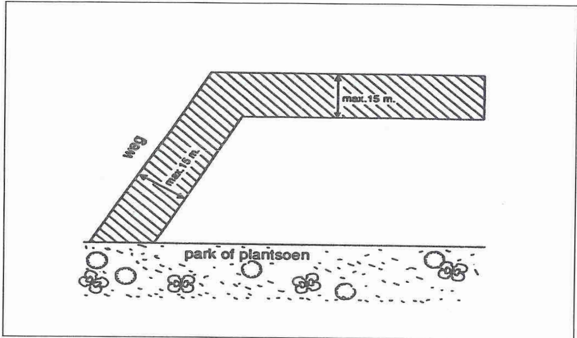
Figuur 10 Ligging van de achtergevelrooilijn (artikel 2.5.11, eerste lid, onder e)
