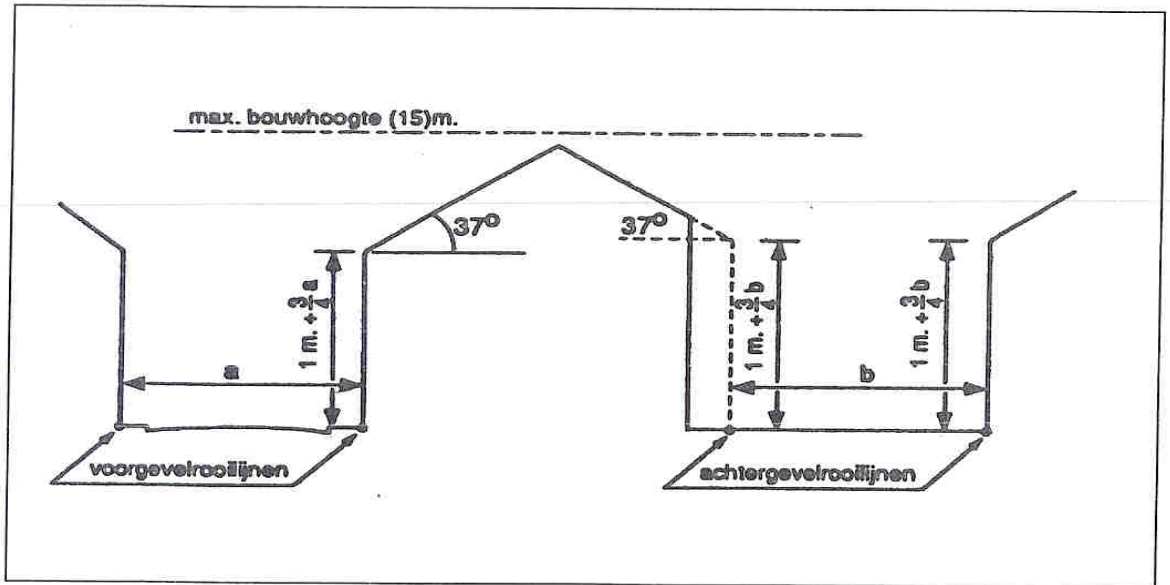
in voor- en achtergevelrooilijn en daartussen. Maximum bouwhoogte (artikelen 2.5.20, 2.5.21, 2.5.23 en 2.5.25). Buiten de bebouwde kom
