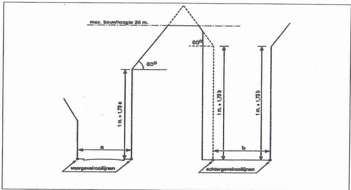
Figuur 14 Bouwhoogte in voor- en achtergevelrooilijn en daartussen. Maximum bouwhoogte (artikelen 2.5.20, 2.5.21, 2.5.23 en 2.5.24, alternatief 2). Binnen grootstedelijke
