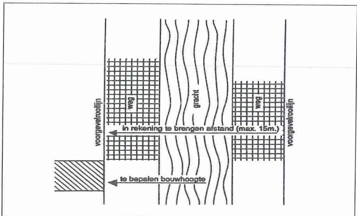
Figuur 14 Bouwhoogte in voor- en achtergevelrooilijn en daartussen. Maximum bouwhoogte (artikelen 2.5.20, 2.5.21, 2.5.23 en 2.5.24, alternatief 2). Binnen grootstedelijke
