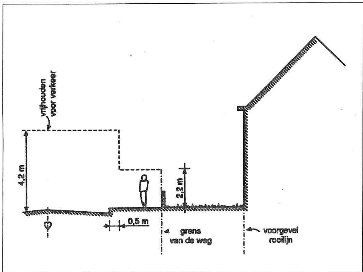
Figuur 1 Voor verkeer vrij te houden hoogten (artikel 2.5.11, eerste lid, onder c)
