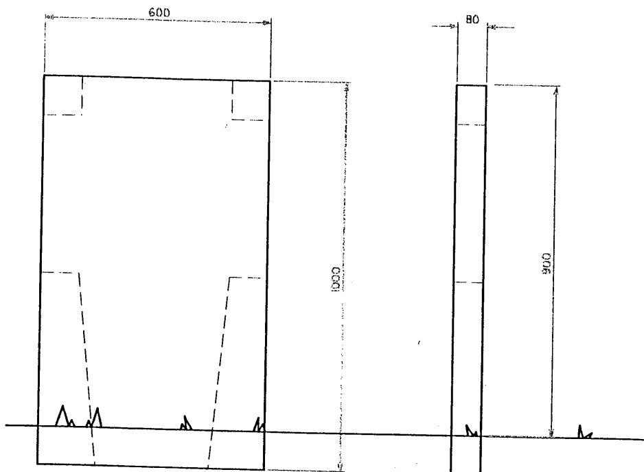
Vooranzicht schaal 1:10
