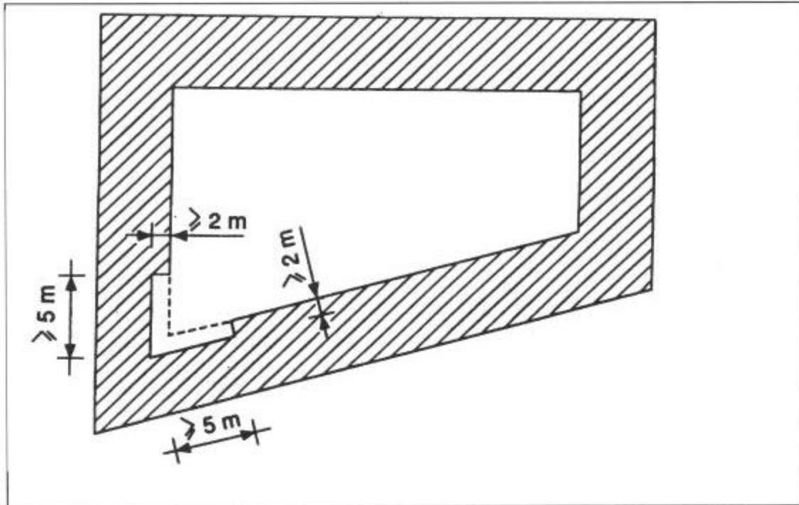
Figuur 11: Teruglegging met het oog op de daglicht toetreding van achtergevelrooilijn die een scherpe hoek met elkaar vormen (ingevolge artikel 2.3.8, lid 2)
