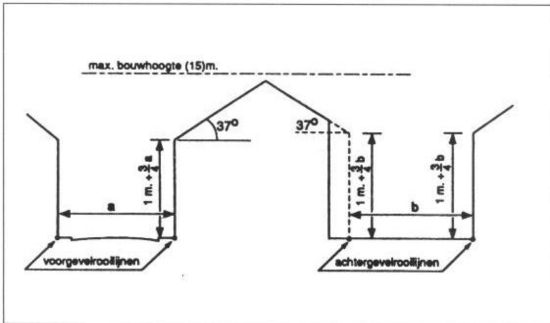
Figuur 13: Bouwhoogte in voor- en achtergevelrooilijn en daartussen. Maximum bouwhoogte (artikelen 2.3.17, 2.3.18, 2.3.20 en 2.3.22). Buiten de bebouwde kom.
