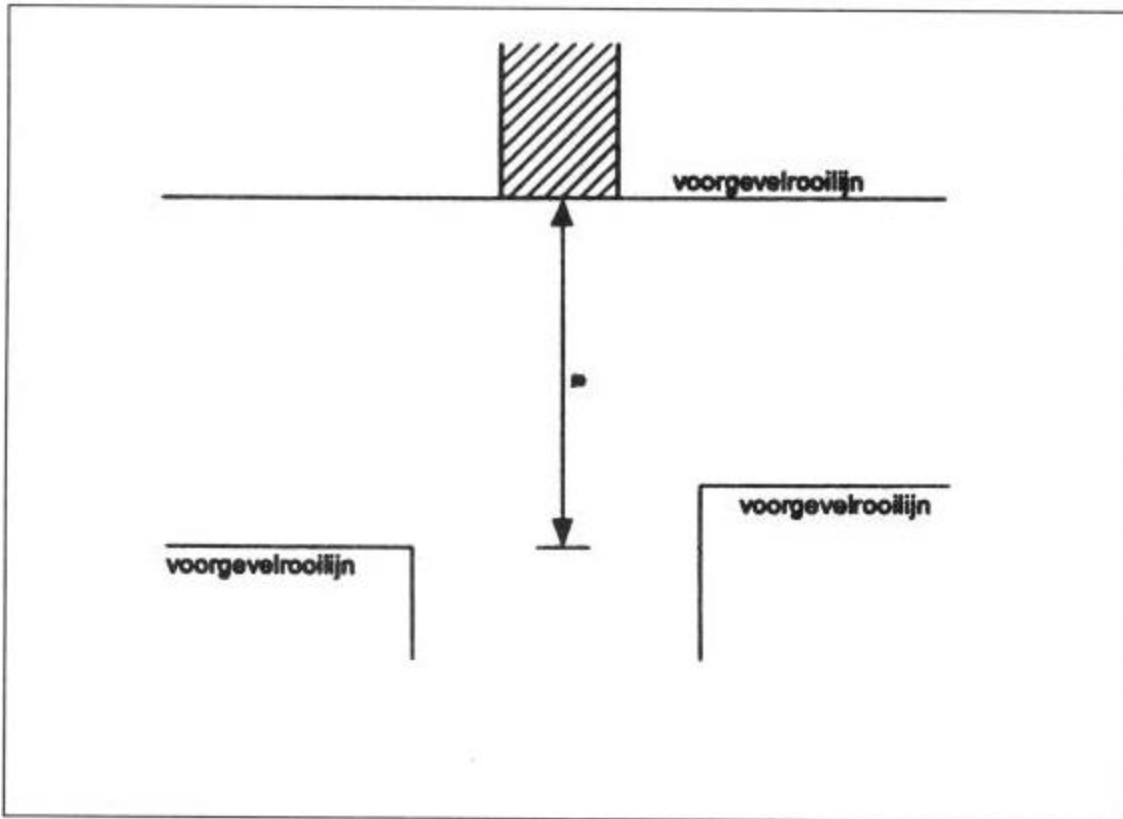
Figuur 15: Bouwhoogte in de voorgevelrooilijn (artikel 2.3.17, derde lid, tweede alinea)
