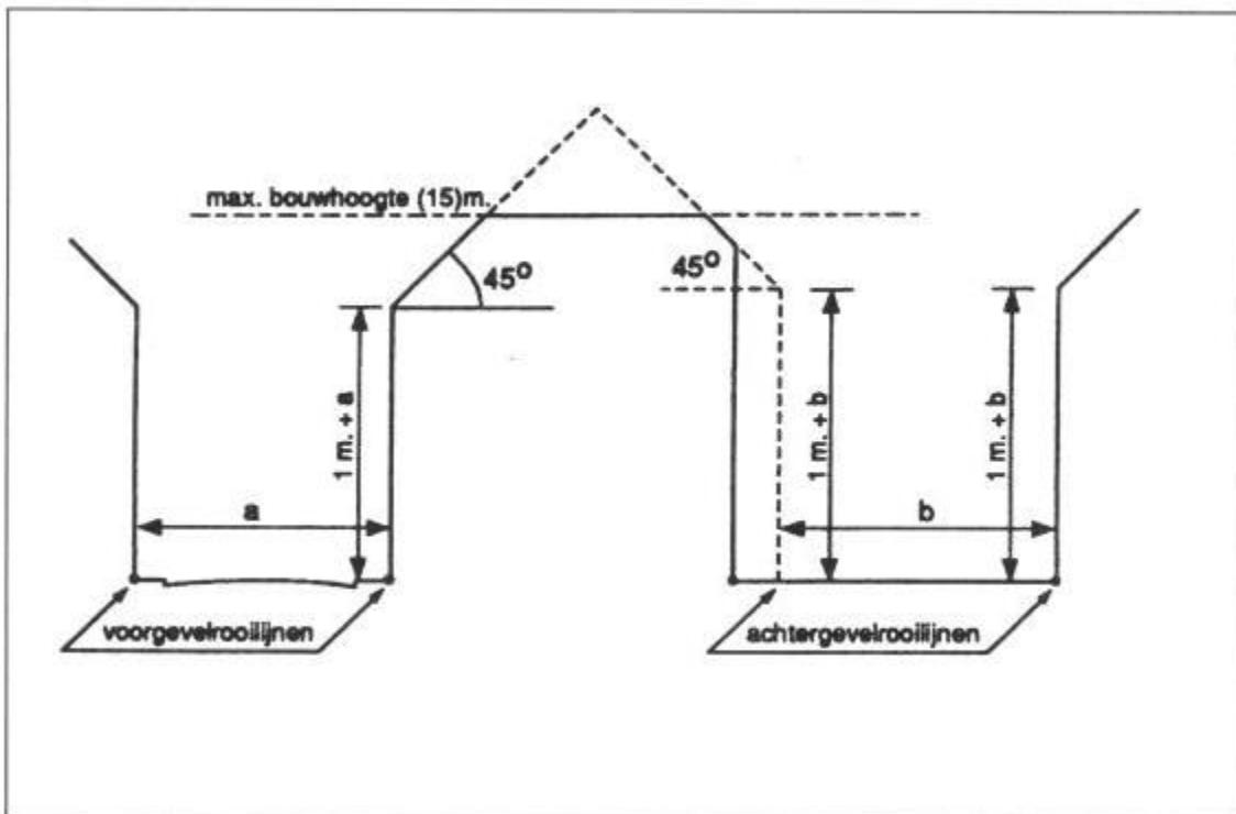
Figuur 12: Bouwhoogte in voor- en achtergevelrooilijn en daartussen. Maximum bouwhoogte (artikelen 2.3.17, 2.3.18, 2.3.20 en 2.3.22). Binnen de bebouwde kom.
