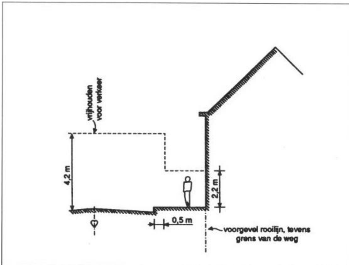
Figuur 2: Voor verkeer vrij te houden hoogten (artikelen 2.3.4 en 2.3.5)
