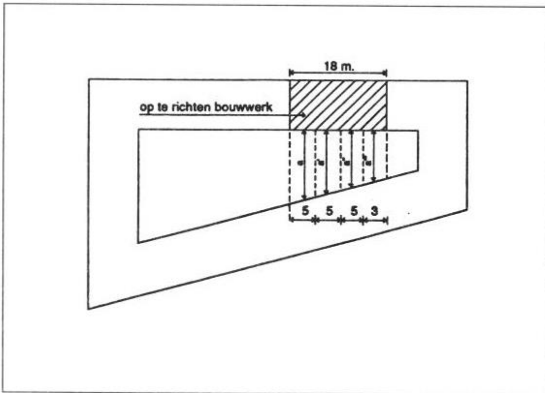
Figuur 16: Bouwhoogte in de achtergevelrooilijn (artikel 2.3.18, tweede lid, eerste alinea)
