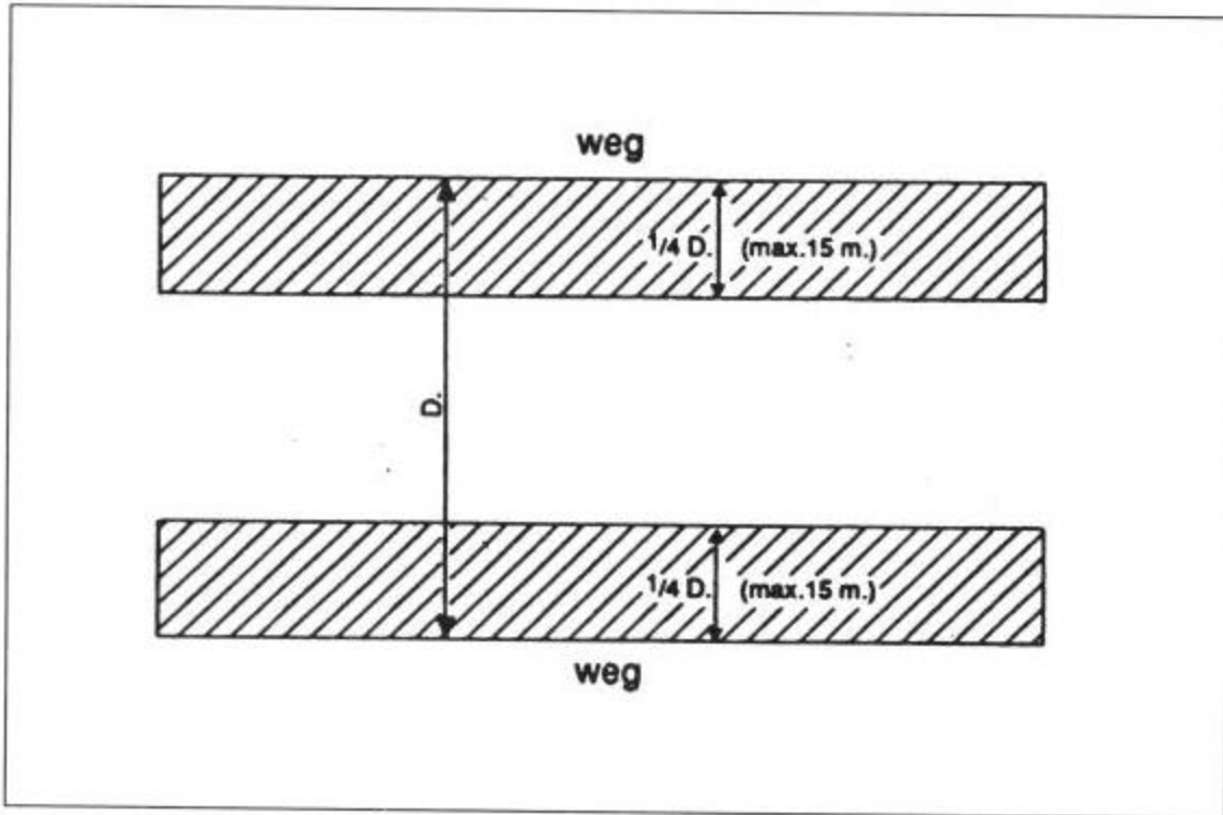
Figuur 9: Ligging van de achtergevelrooilijn (artikel 2.3.8, eerste lid, onder d)
