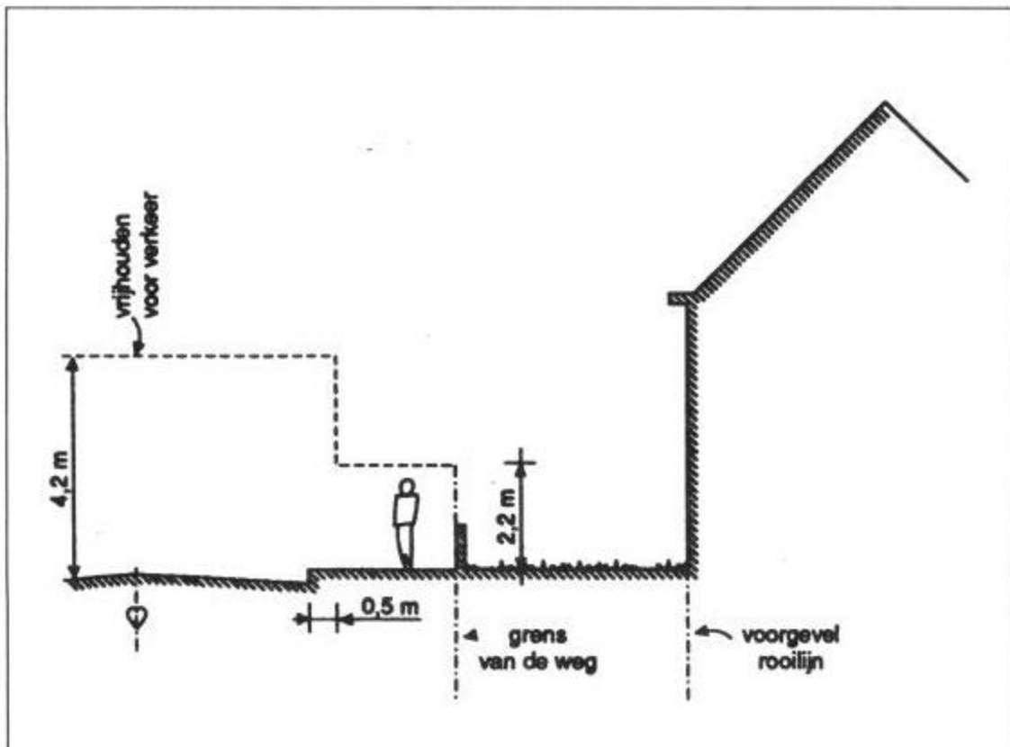
Figuur 1: Voor verkeer vrij te houden hoogten (artikelen 2.3.4 en 2.3.5)
