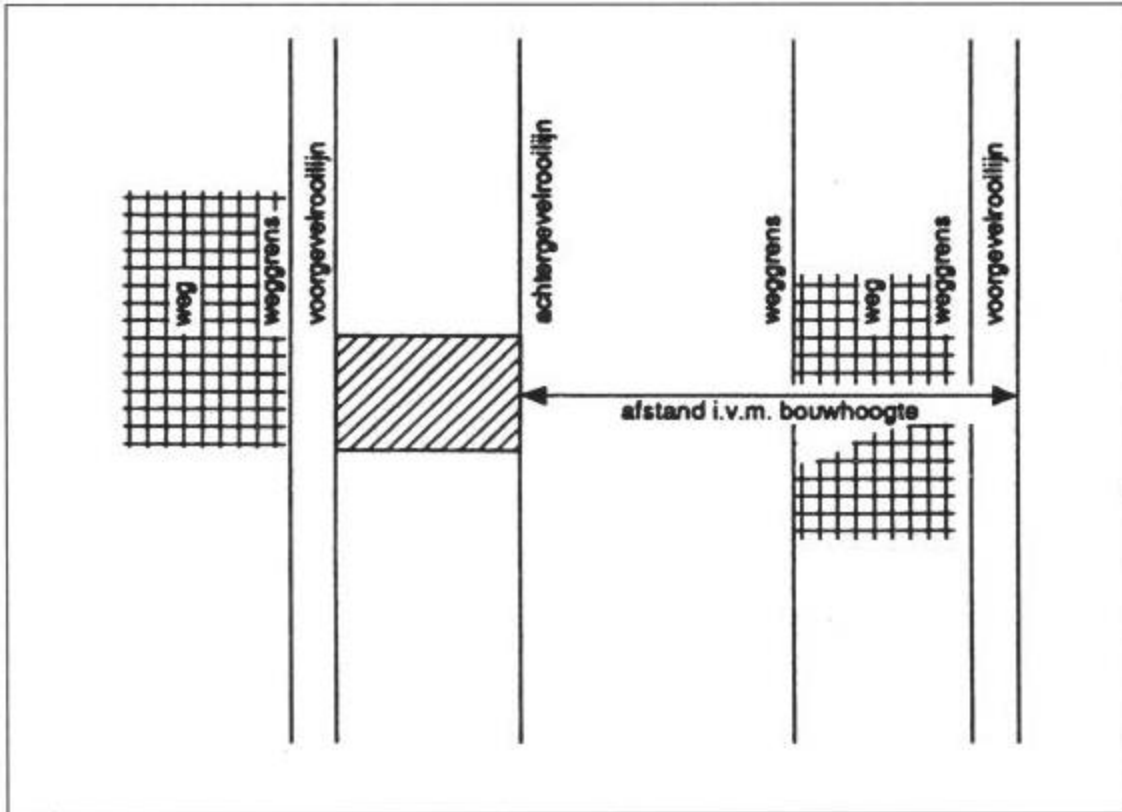
Figuur 17: Bouwhoogte in de achtergevelrooilijn (artikel 2.3.17, tweede lid, tweede alinea)
