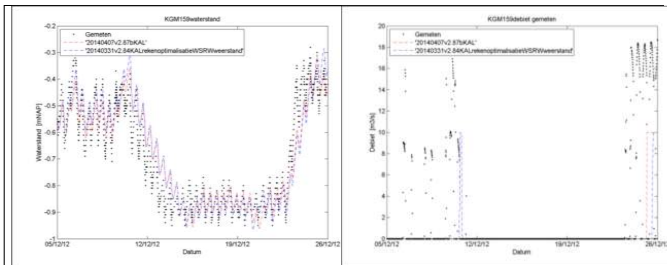
Figuur 7-37. Gesimuleerde waterstand bij uitwateringspunt Braakman (links) en verpompte debiet (rechts).
