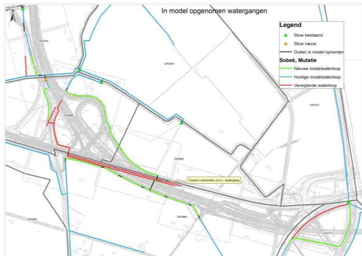
Figuur 7-66. Modelwaterlopen rondom Sluiskiltunnel en N61.
