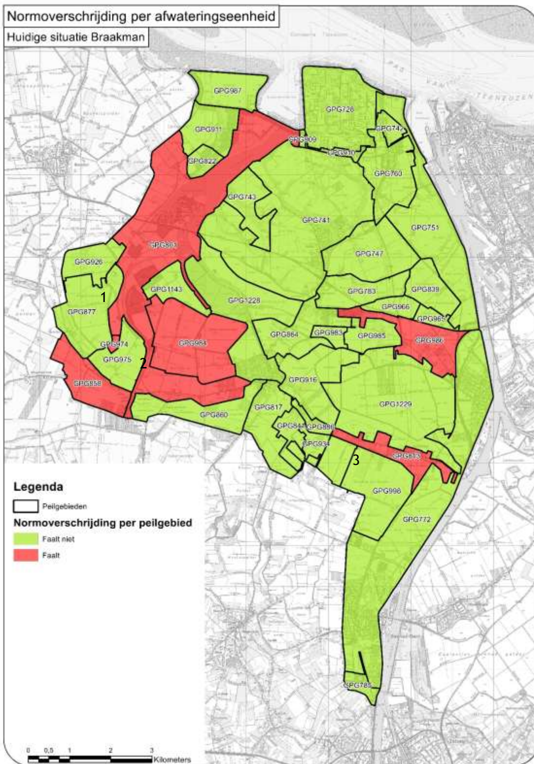
Figuur 5-6. Normoverschrijding per afwateringseenheid voor huidige situatie.
