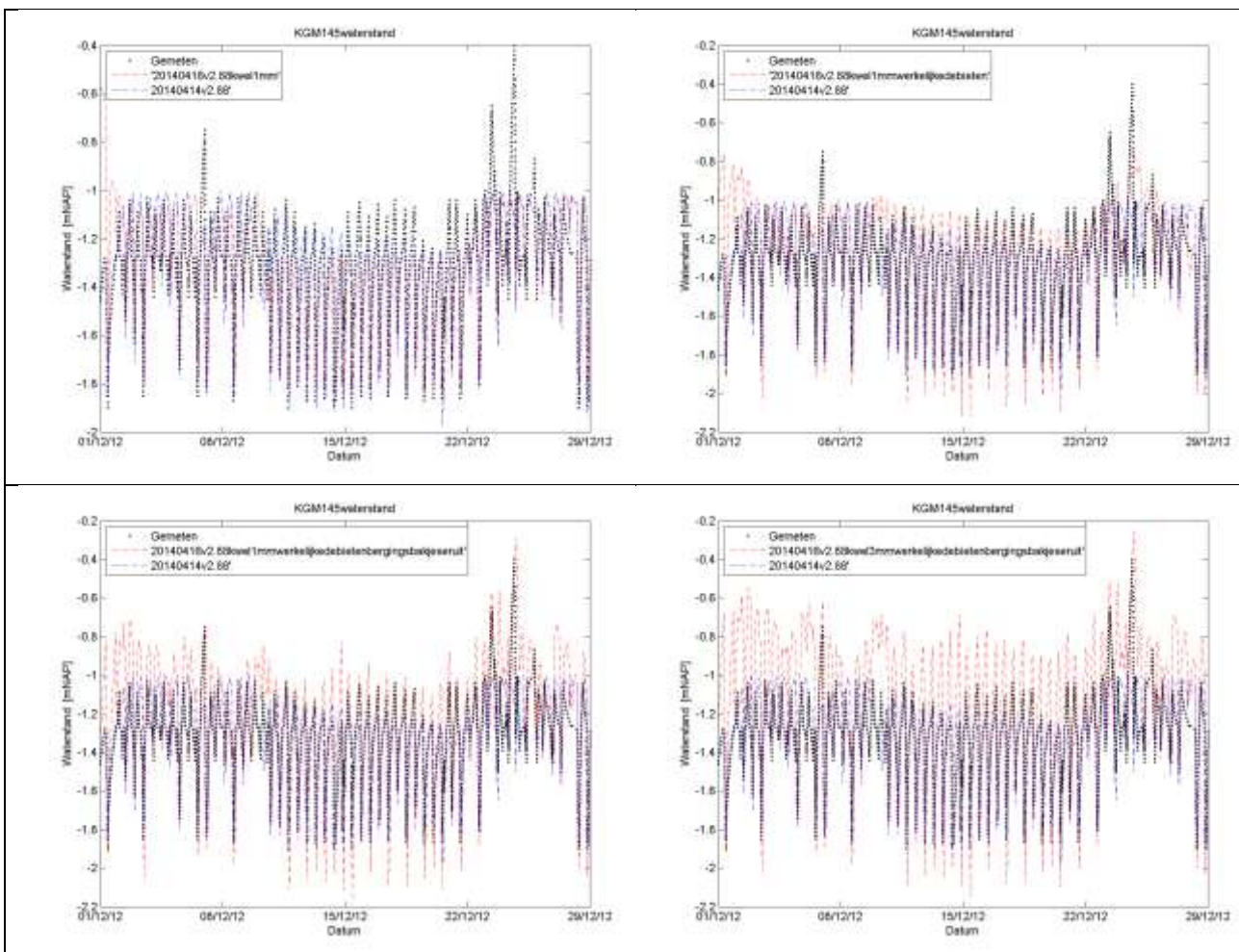
Figuur 7-34. Linksboven = kwel 1 mm/dag, zonder geblokkeerde uitwatering, rechtsboven = kwel 1 mm/dag met geblokkeerde uitwatering, linksonder = kwel 1 mm/dag met geblokkeerde uitwatering en zonder bergingsbakjes en rechtsonder = kwel 3 mm/dag met geblokkeerde uitwatering en zonder bergingsbakjes.
