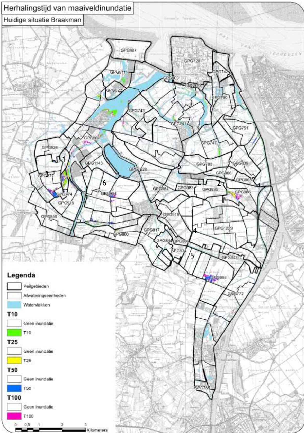
Figuur 5-4. Herhalingstijd van maaiveldinundatie bij huidige situatie.
