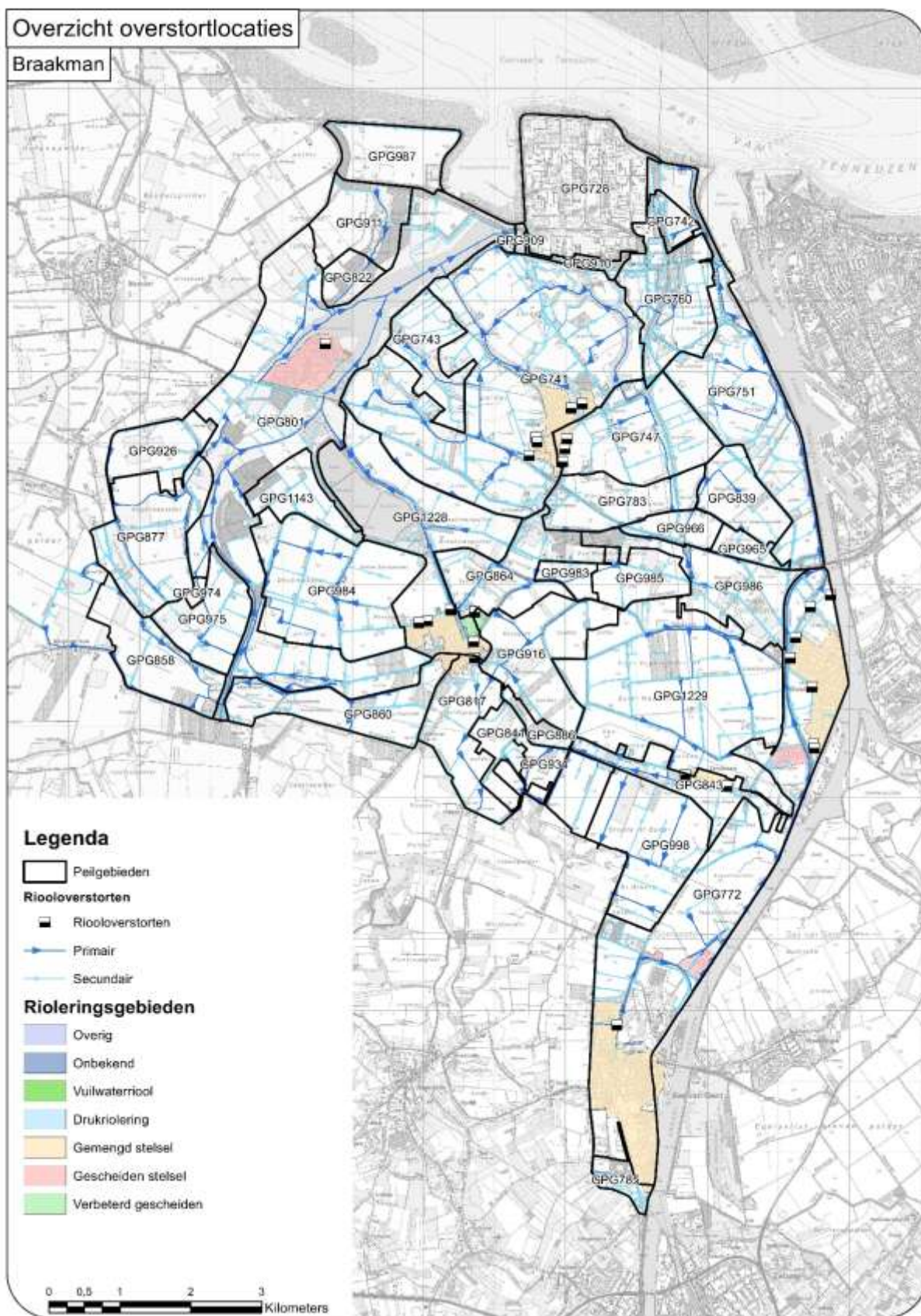
Figuur 2-15. Overzicht overstortlocaties.
