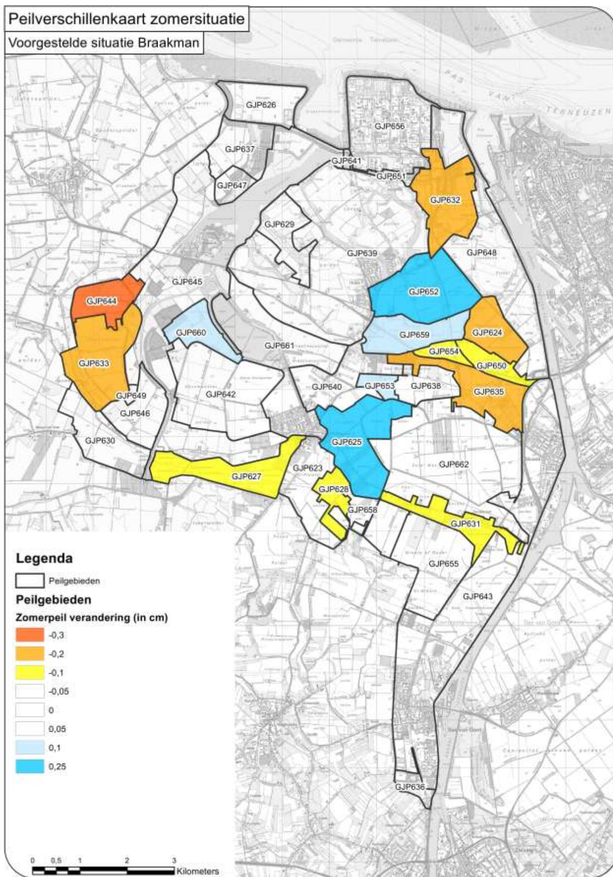
Figuur 6-13. Peilverandering in de zomer.
