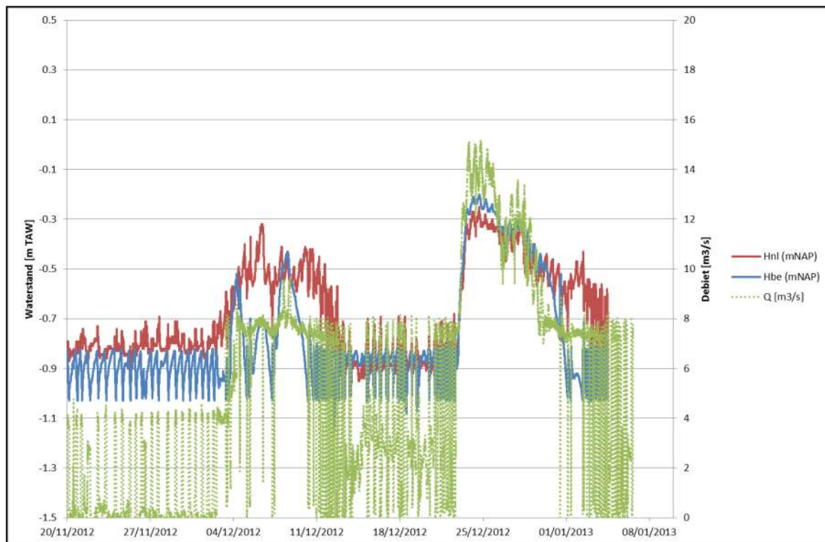
Figuur 7-69. Meetgegevens beschikbaar vanuit Hydronet.be (gemaal Isabella).
