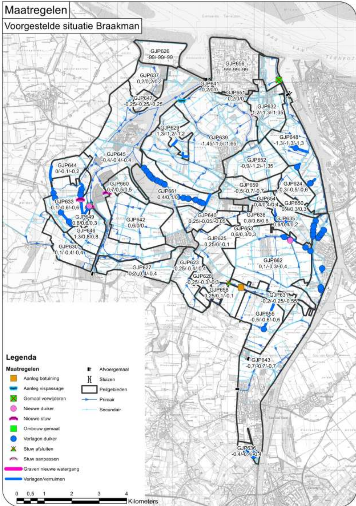
Figuur 6-4. Maatregelen t.b.v peilbeheer onder normale omstandigheden.
