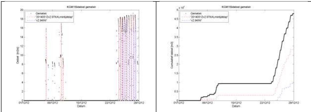
Figuur 7-48. Debieten gemaal Braakman.
