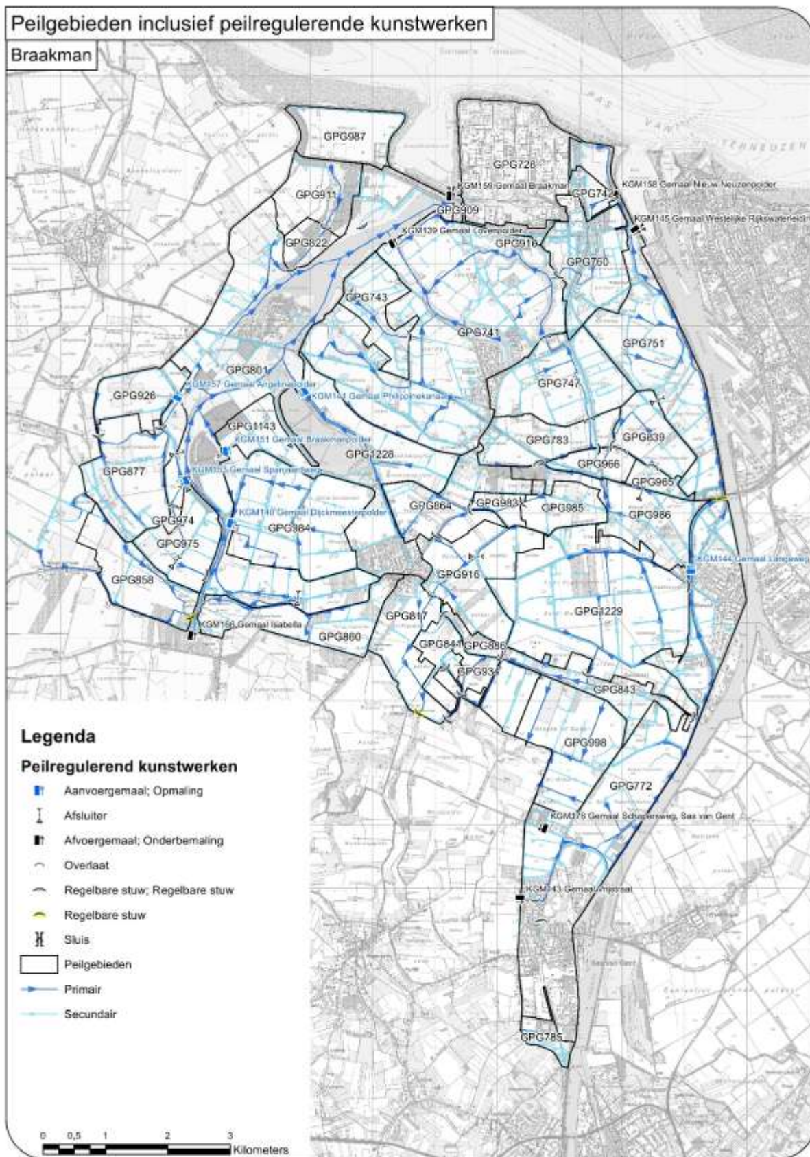
Figuur 2-10. Peilgebieden inclusief peilregulerende kunstwerken.
