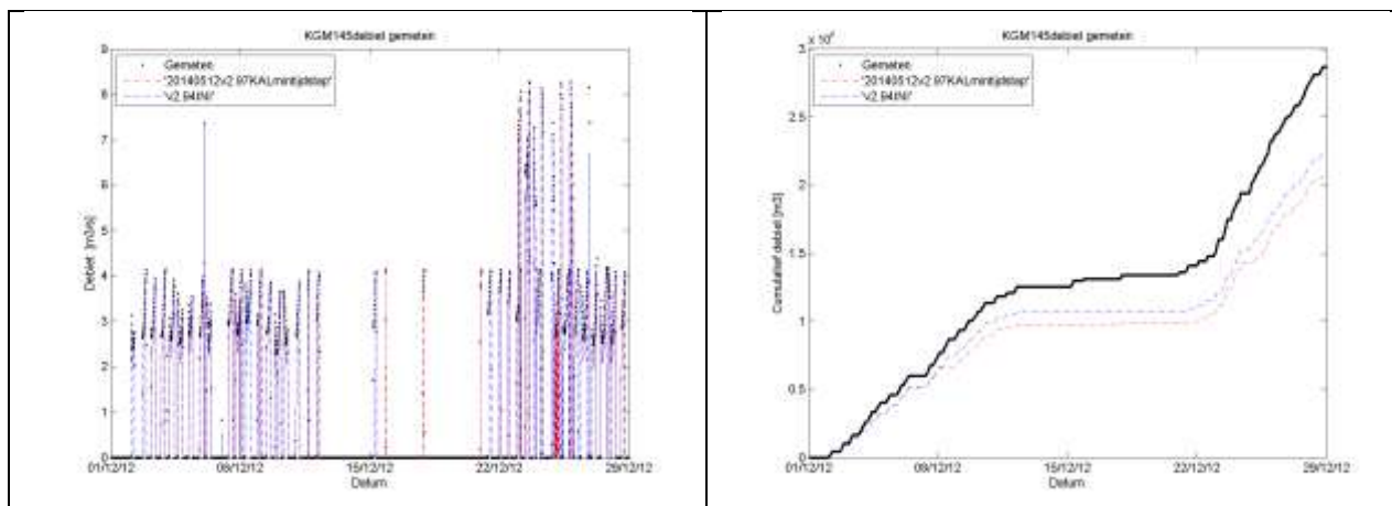
Figuur 7-46. Debietsen gemaal Westelijke Rijkswaterleiding.
