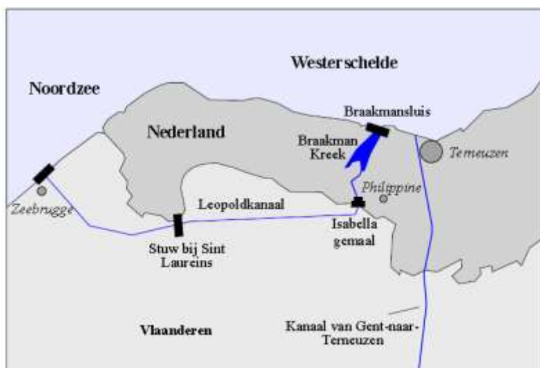
Figuur 2-2. Schematische weergave watersysteem Leopoldkanaal-Braakman (Bron: Hydrologic, 2007).
