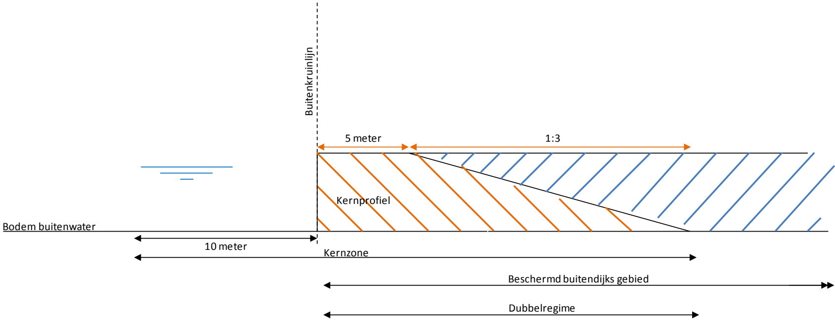
Figuur Zonering waterkering met damwandconstructie
