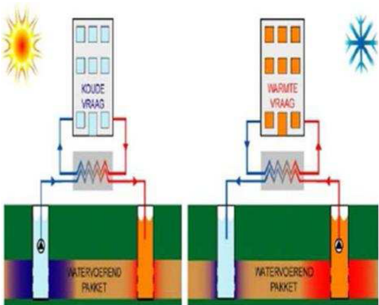
Afbeelding 1. Open bodemenergiesysteem
