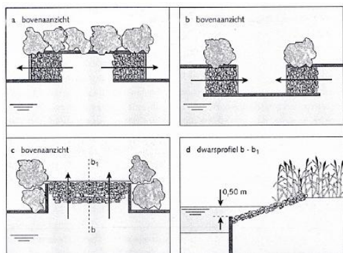
Figuur 6.4 Drie basis varianten voor fauna-uitstapplaatsen; tekening "d" betreft een dwarsprofiel van variant "c" (bron: RWS).
