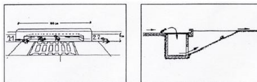
Figuur 6.6 Enkele voorzieningen voor amfibieën bij wegioleringssystemen (bron: RWS).
