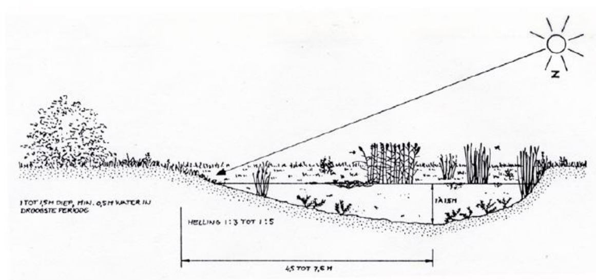
Figuur 2 Principe-profiel poel (bron: Landschapsbeheer Nederland, 1998).
